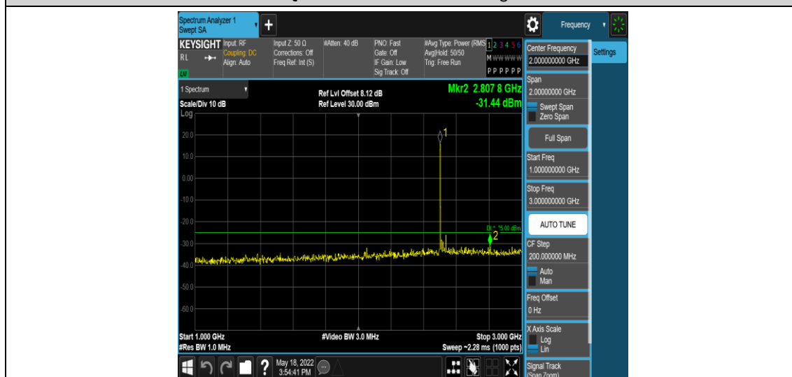
Band7-20MHz-QPSK-20850-1RB#0-Range4:1000~3000MHz
