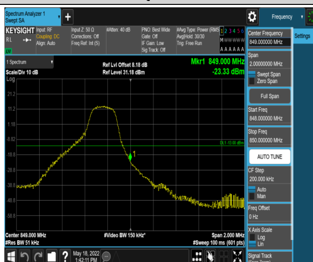
Band5-3MHz-QPSK-20635-1RB#14
