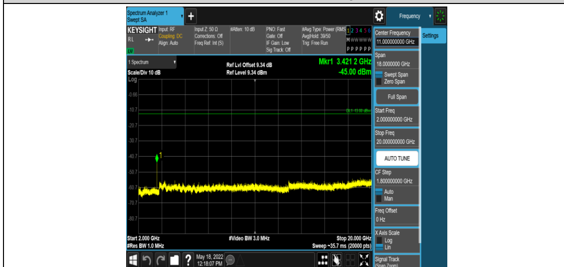
Band4-10MHz-QPSK-20000-1RB#0-Range5:2000~20000MHz
