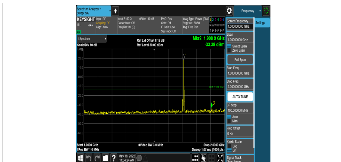
Band4-3MHz-QPSK-19965-1RB#0-Range4:1000~2000MHz
