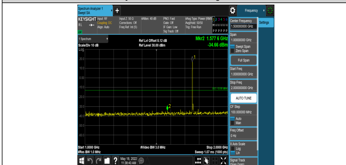
Band4-3MHz-QPSK-20385-1RB#0-Range4:1000~2000MHz
