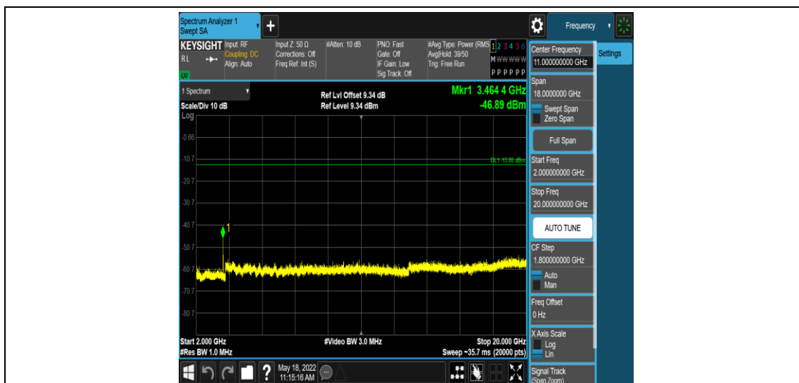
Band4-1.4MHz-QPSK-20175-1RB#0-Range5:2000~20000MHz
