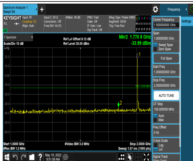
Band2-5MHz-16QAM-19175-1RB#0-Range4:1000~2000MHz
