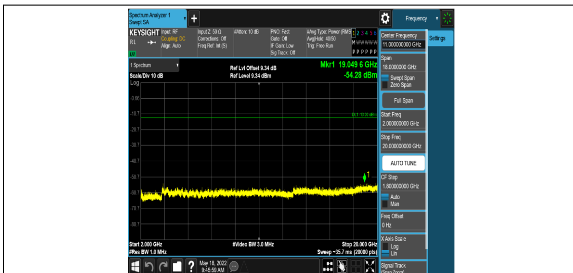
Band2-5MHz-QPSK-18625-1RB#0-Range5:2000~20000MHz
