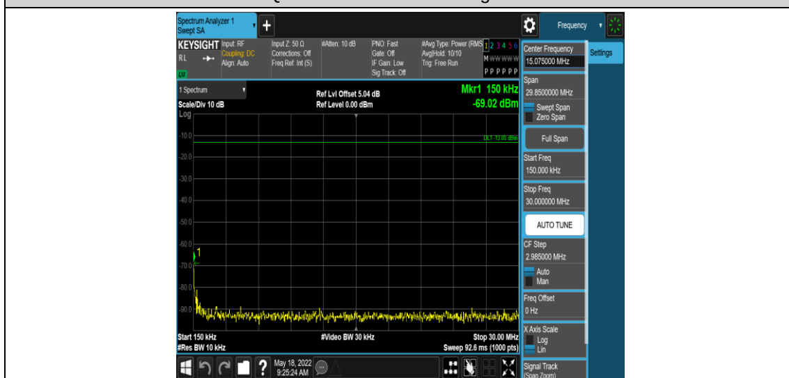
Band2-3MHz-QPSK-18900-1RB#0-Range2:0.15~30MHz
