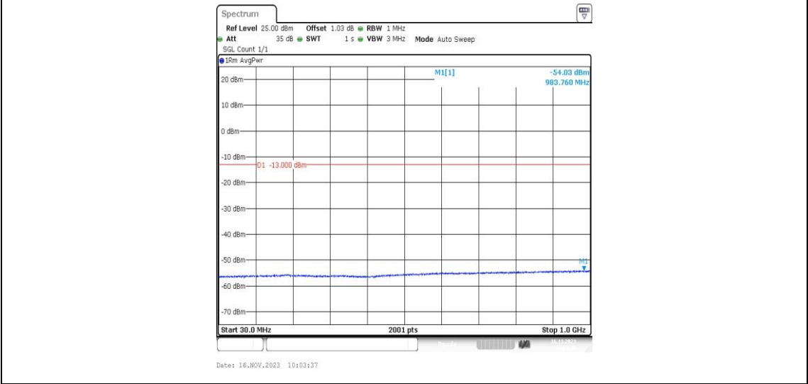
Band4-1312-30-1000MHz-PASS
