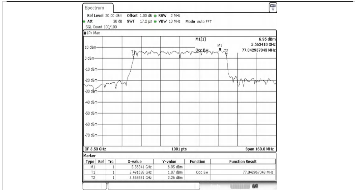
11AC80SISO-Ant1-5530
