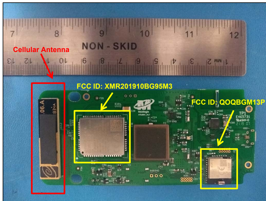
EUT PCB Top Side
