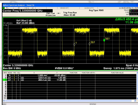
IEEE 802.11n_20MHz_Channel 64
