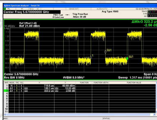
IEEE 802.11n_40MHz_Channel 134
