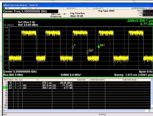
IEEE 802.11ac_20MHz_Channel 100
