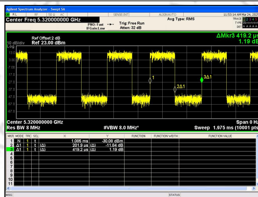
IEEE 802.11ac_20MHz_Channel 64
