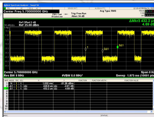
IEEE 802.11n_20MHz_Channel 140
