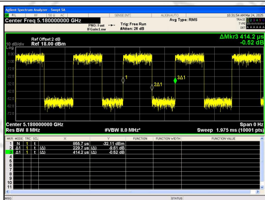
IEEE 802.11n_20MHz_Channel 36
