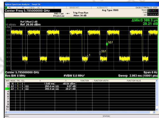
IEEE 802.11a_20MHz_Channel 157
