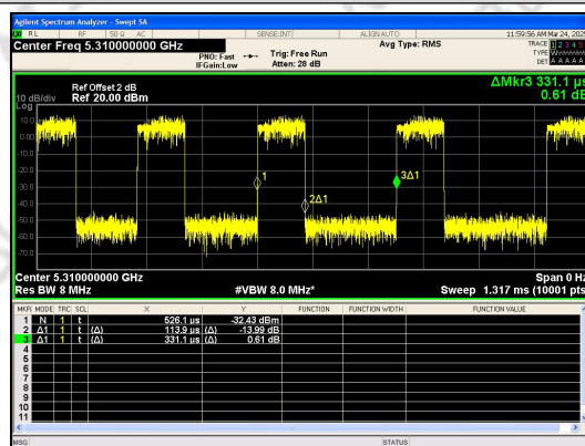
IEEE 802.11ac_40MHz_Channel 62
