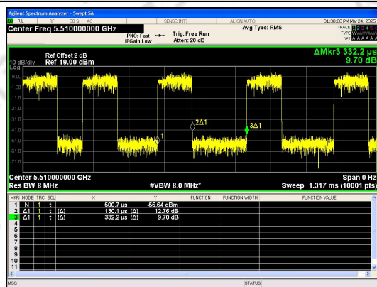
IEEE 802.11n_40MHz_Channel 102
