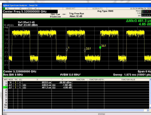
IEEE 802.11a_20MHz_Channel 64
