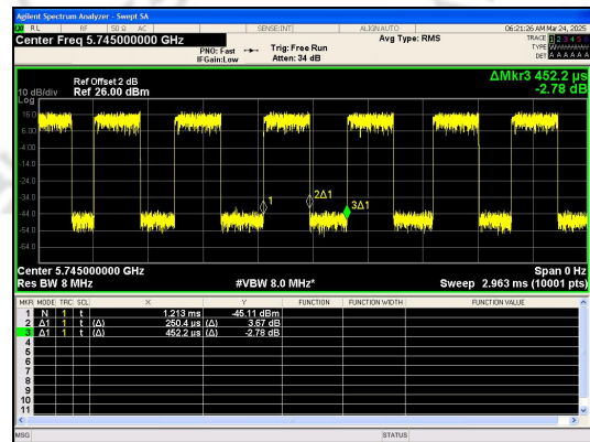
IEEE 802.11a_20MHz_Channel 149
