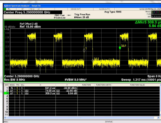
IEEE 802.11ac_80MHz_Channel 58
