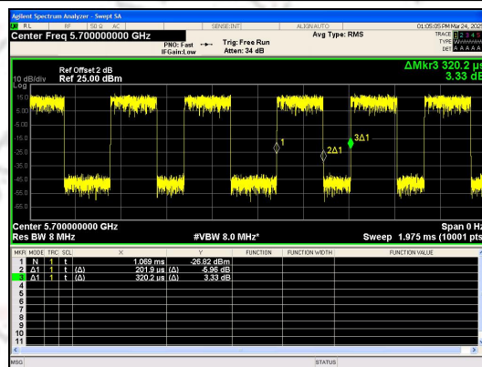
IEEE 802.11ac_20MHz_Channel 140
