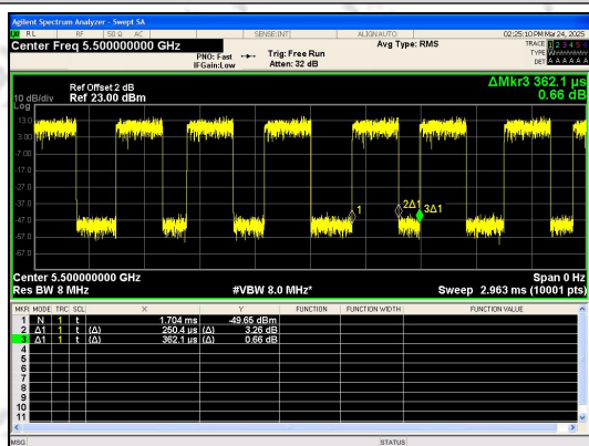
IEEE 802.11a_20MHz_Channel 100
