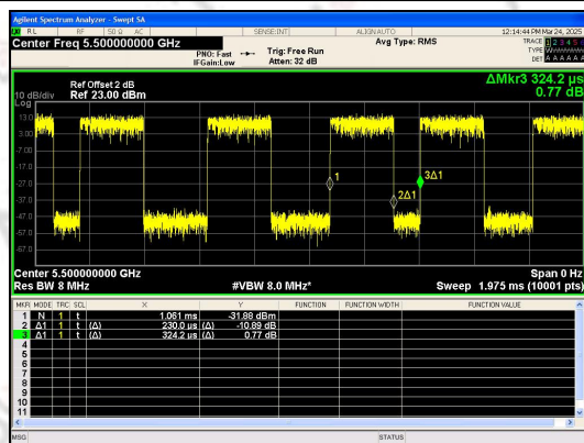
IEEE 802.11n_20MHz_Channel 100
