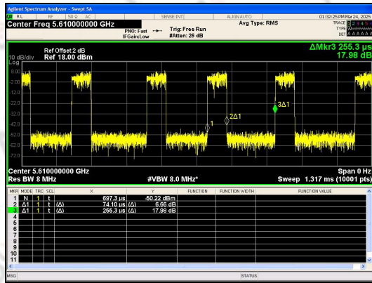
IEEE 802.11ac_80MHz_Channel 122
