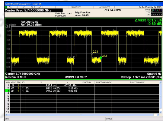
IEEE 802.11n_20MHz_Channel 149
