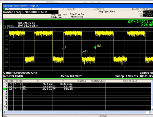
IEEE 802.11a_20MHz_Channel 140
