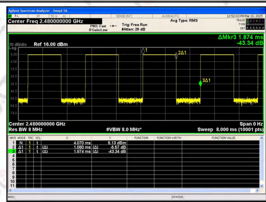
BLE 2M_Channel 39
