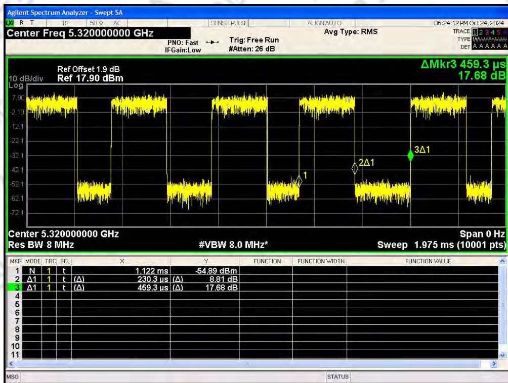
IEEE 802.11n_20MHz_Channel 64
