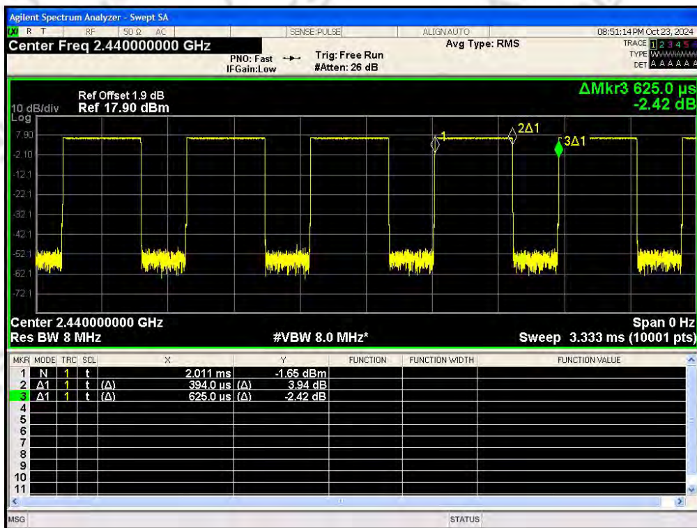
BLE 1M_Channel 19
