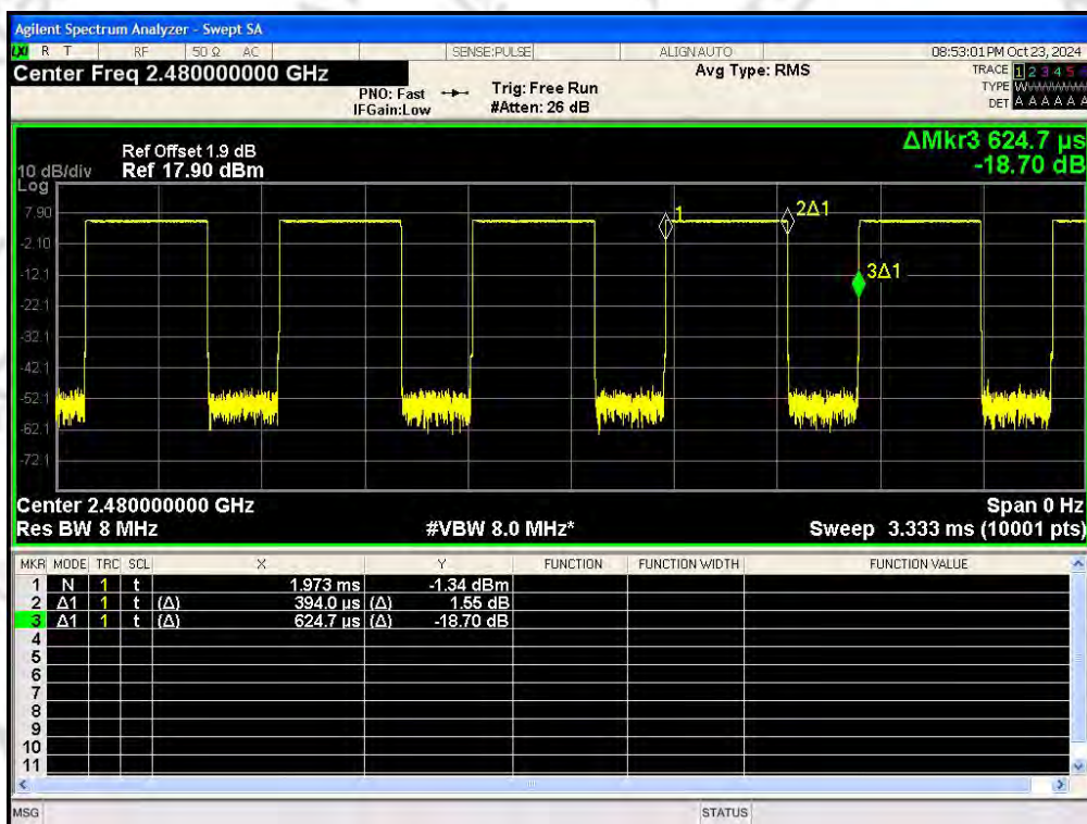
BLE 1M_Channel 39
