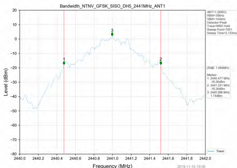
GFSK_2441MHz_DH5_SISO_ANT1
