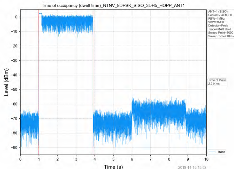
8DPSK_Hopping_3DH5_SISO_ANT1
