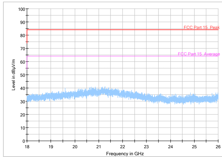
Fig.77 18GHz~26GHz
