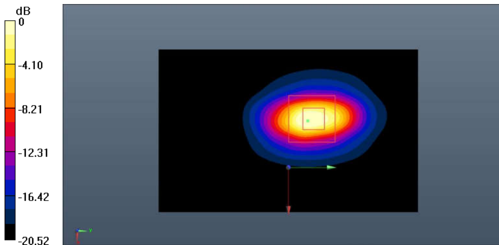
Fig.B.5. Validation 2300MHz 250mW
