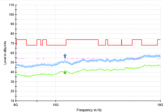
RSE-11N(40M)-CH54-8GHz-18GHz
