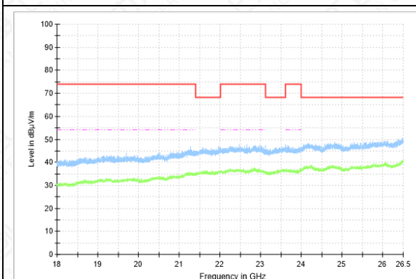
RSE-11N-CH56-18GHz-26.5GHz
