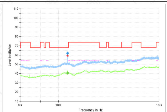
RSE-11N-CH56-8GHz-18GHz
