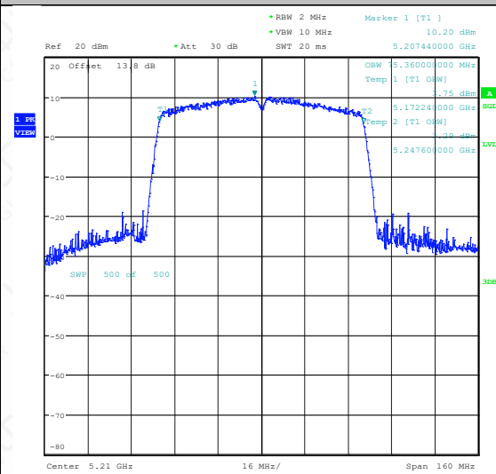
11AC80SISO-Ant1-5210
