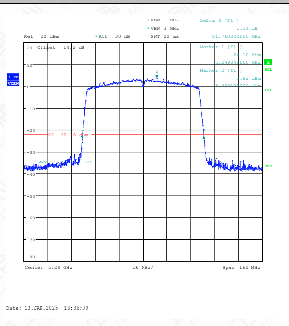
11AC80SISO-Ant1-5290
