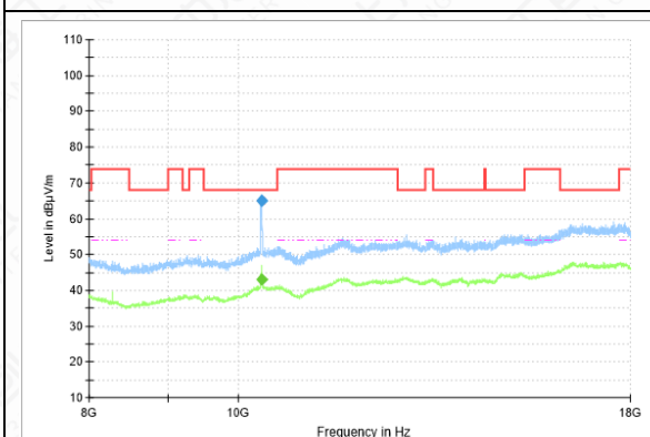
RSE-11N-CH36-8GHz-18GHz
