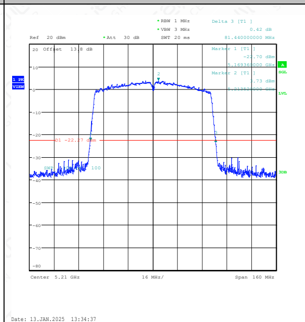
11AC80SISO-Ant1-5210
