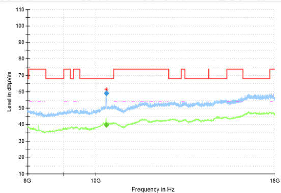
RSE-11AC-CH36-8GHz-18GHz
