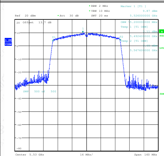
11AC80SISO-Ant1-5530
