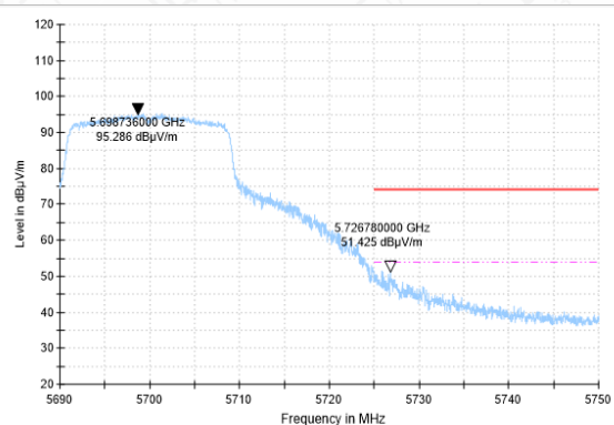
BANDEGE-11AC-CH140-AV
