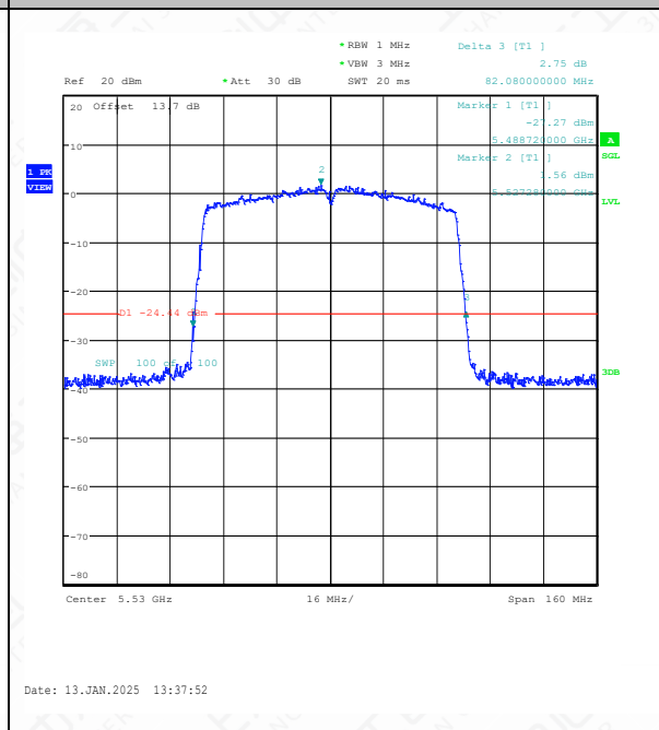
11AC80SISO-Ant1-5530
