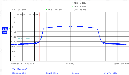
11N40SISO-Ant1-5270-PASS
