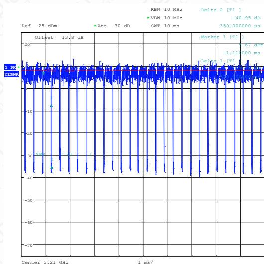
NTNV-11AC80SISO-Ant1-5210
