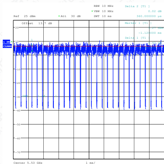
NTNV-11AC80SISO-Ant1-5530
