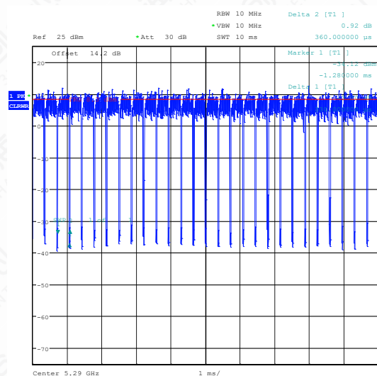
NTNV-11AC80SISO-Ant1-5290
