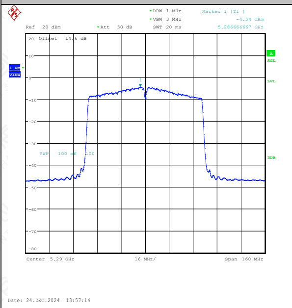
11AC80SISO-Ant1-5290-PASS
