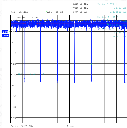
NTNV-11A-Ant1-5280
