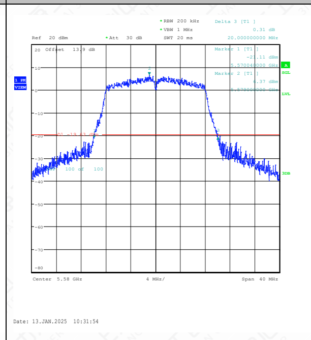
11A-Ant1-5580
