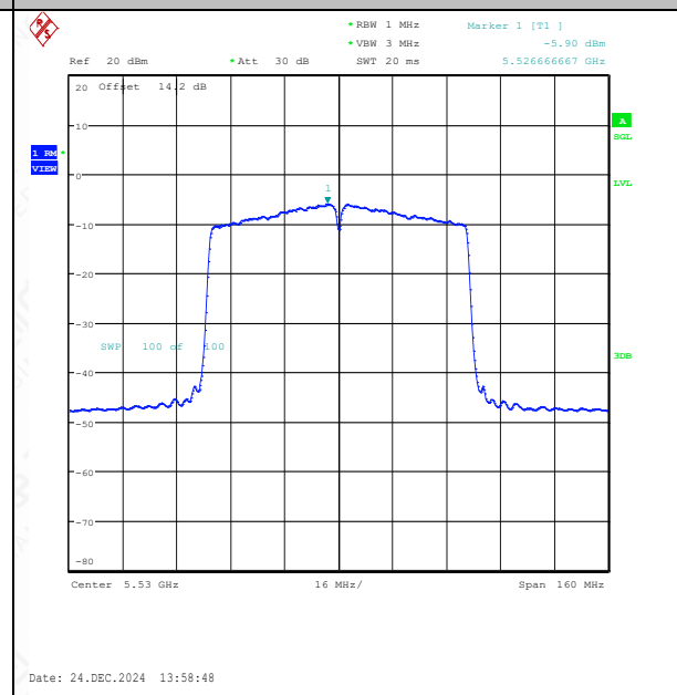
11AC80SISO-Ant1-5530-PASS
