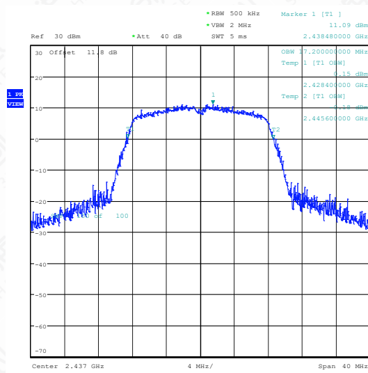
11G-Ant1-2437
