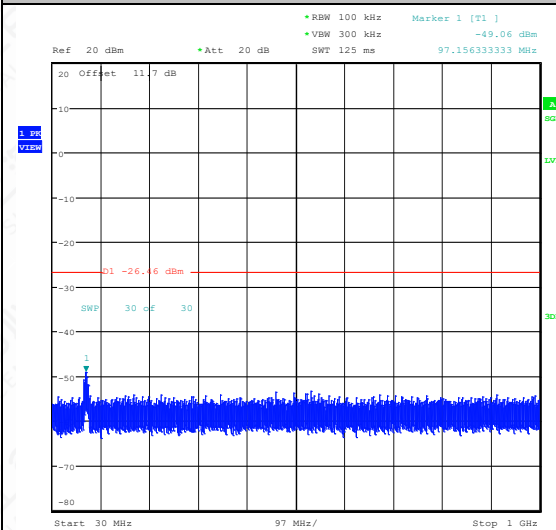
11G-Ant1-2412-30~1000-PASS
