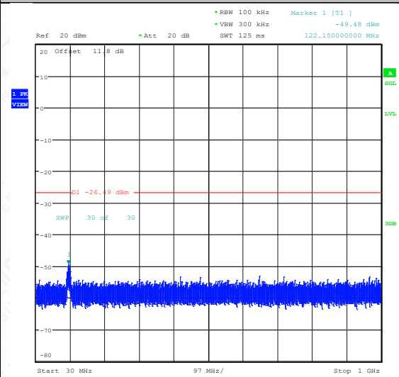
11G-Ant1-2437-30~1000-PASS
