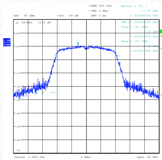
11G-Ant1-2462
