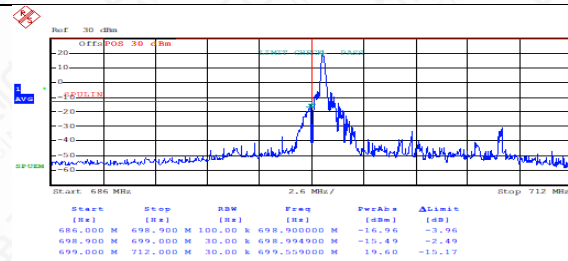
FDD12LowRange_10MHz_QPSK_1RB_LowRange
