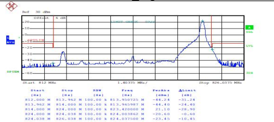
FDD26(Part 90)_Low_10MHz_QPSK_1RB high
