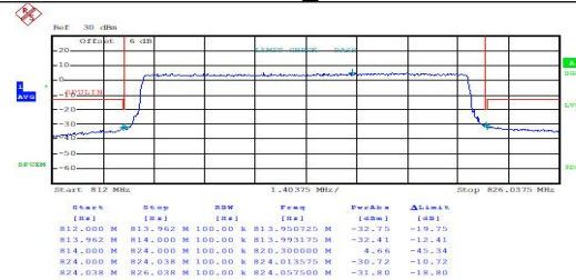
FDD26(Part 90)_Low_10MHz_QPSK_FullRB Low
