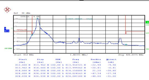
FDD26(Part 90)Low_10MHz_QPSK_1RB low
