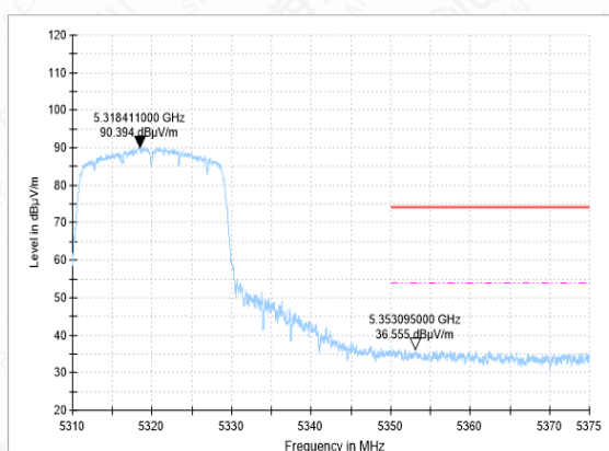
Bandedge-11AC(20M)-CH64-AV
