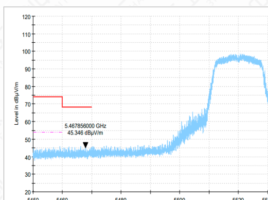
Bandedge-11A-CH104-PK
