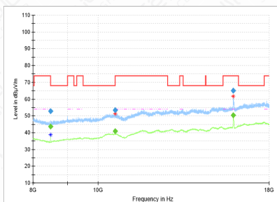
RSE-11N(40M)-CH62-8GHz-18GHz
