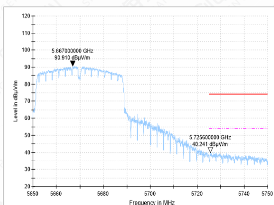
Bandedge-11AC(40M)-CH134-AV
