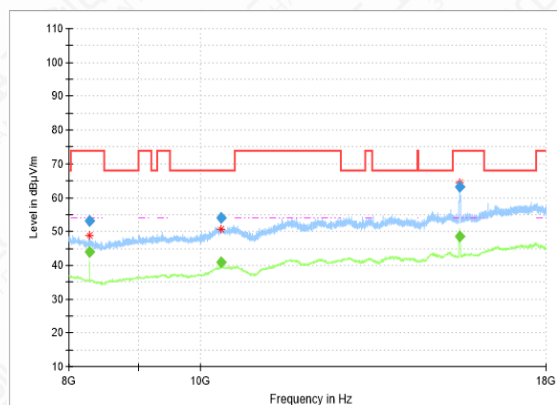
RSE-11N(20M)-CH36-8GHz-18GHz
