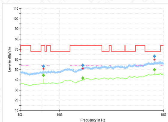
RSE-11A-CH140-8GHz-18GHz
