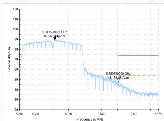
Bandedge-11AC(40M)-CH62-AV
