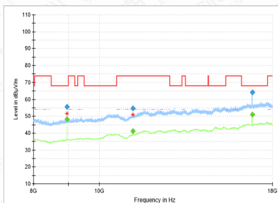
RSE-11N(20M)-CH120-8GHz-18GHz
