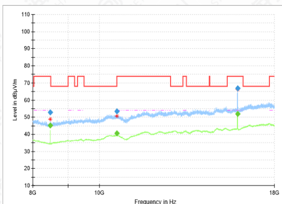
RSE-11N(20M)-CH60-8GHz-18GHz
