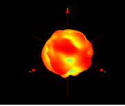
5G(Frequency=5800MHz)
