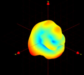
2.4G(Frequency=2500MHz)
