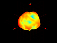
5G(Frequency=5200MHz)
