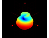
G900/W8(Frequency=940MHz)
