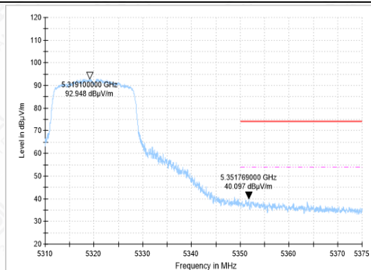
BANDEGE-11A-CH64-AV
