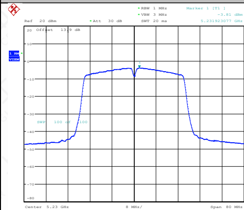
11N40ISO-Ant1-5230-PASS
