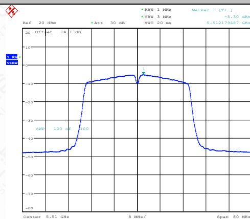
11N40ISO-Ant1-5510-PASS
