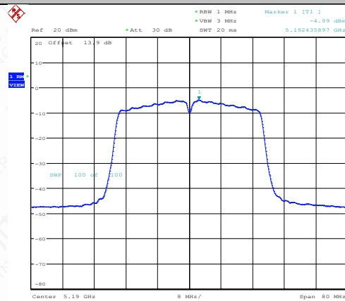
11N40ISO-Ant1-5190-PASS
