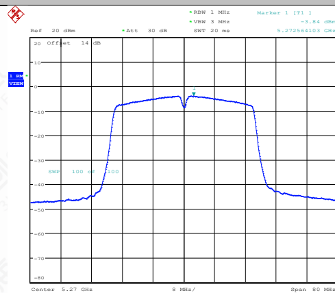
11N40ISO-Ant1-5270-PASS
