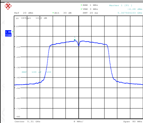
11N40ISO-Ant1-5310-PASS
