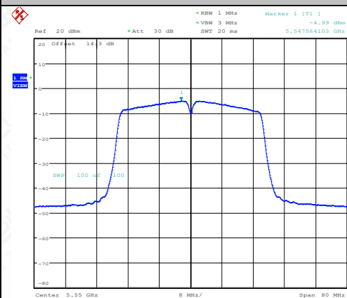
11N40ISO-Ant1-5550-PASS
