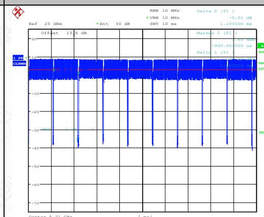
NTNV-11AC80SISO-Ant1-5210
