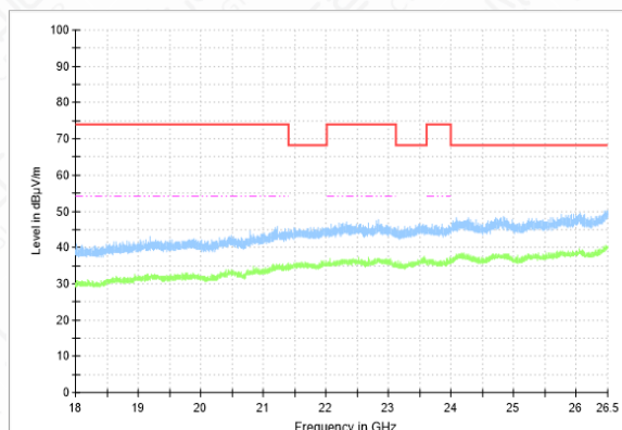
RSE-11AC(40M)-CH151-18GHz-26.5GHz
