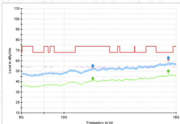
RSE-11AC(40M)-CH151-8GHz-18GHz
