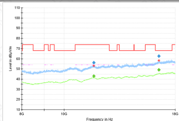
RSE-11AC(80M)-CH155-8GHz-18GHz
