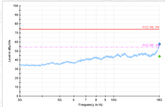
RSE-11G-CH11-3GHz-18GHz
