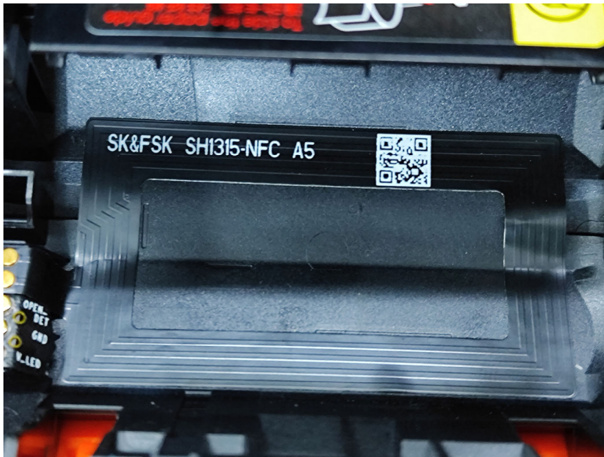
NFC Antenna
