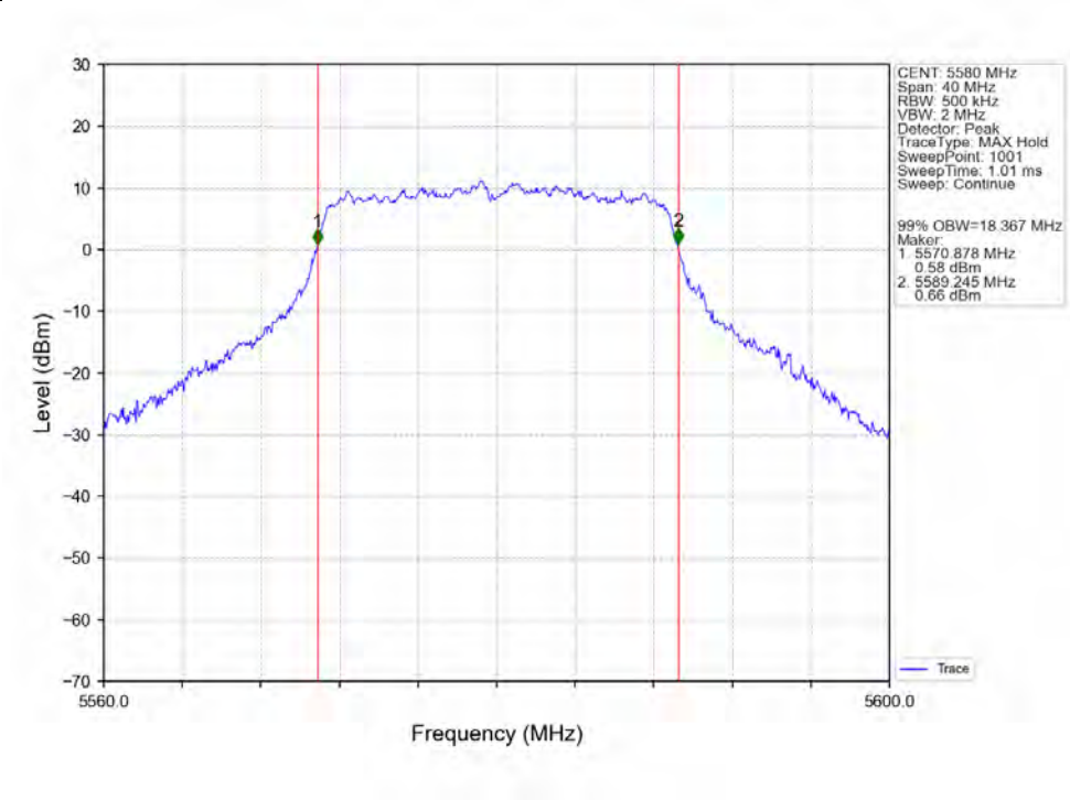
802.11n(HT20)_MCH_5580MHz_Ant1_NTNV
