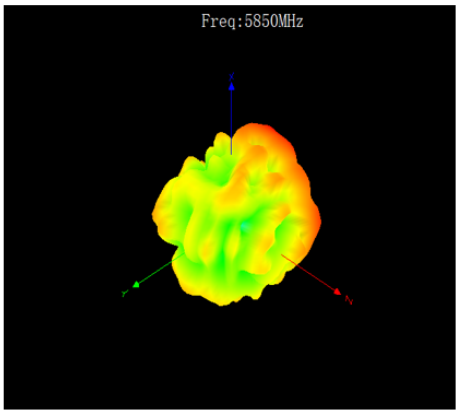
5850MHz
