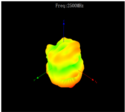
2500MHz
