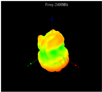
2400MHz
