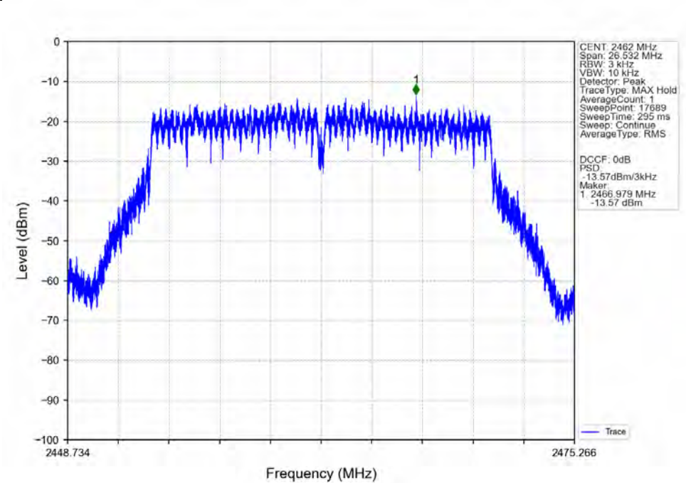
802.11n(HT20)_HCH_2462MHz_Ant1 (SISO)_NTNV
