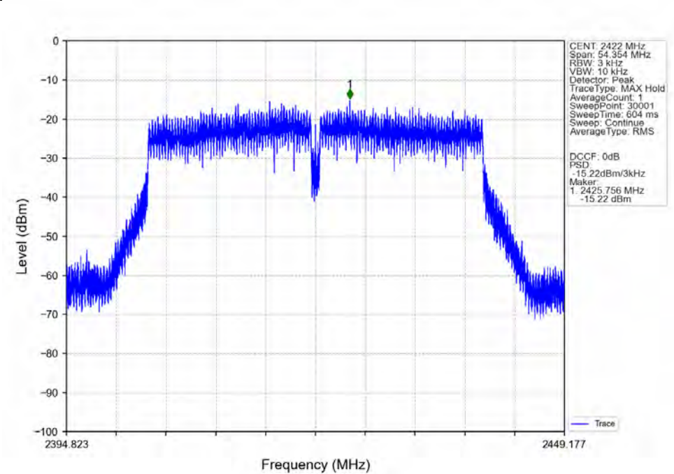
802.11n(HT40)_LCH_2422MHz_Ant1 (SISO)_NTNV
