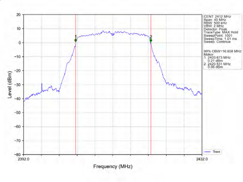
802.11g_LCH_2412MHz_Ant1 (SISO)_NTNV
