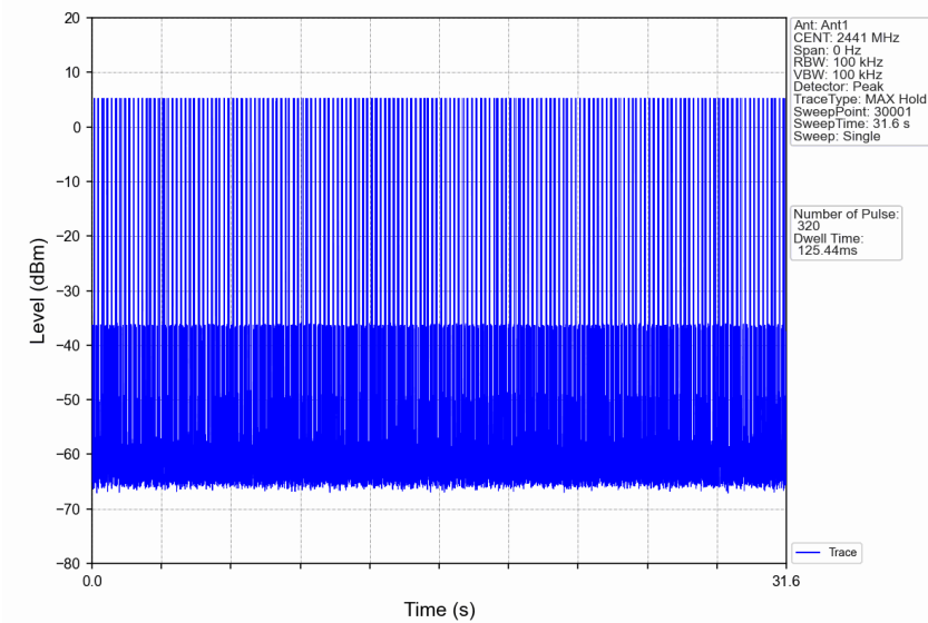
Pi/4DQPSK_2DH1_HOPP_Ant1_NTNV
