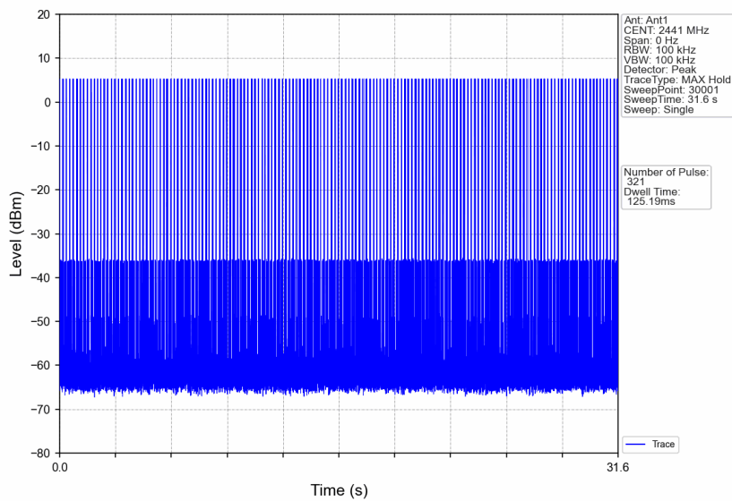
8DPSK_3DH1_HOPP_Ant1_NTNV
