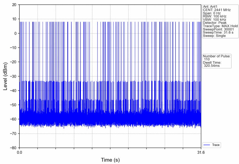
8DPSK_3DH5_HOPP_Ant1_NTNV
