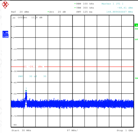
11G-Ant1-2462-30~1000-PASS
