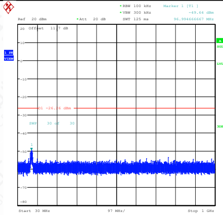
11G-Ant1-2412-30~1000-PASS
