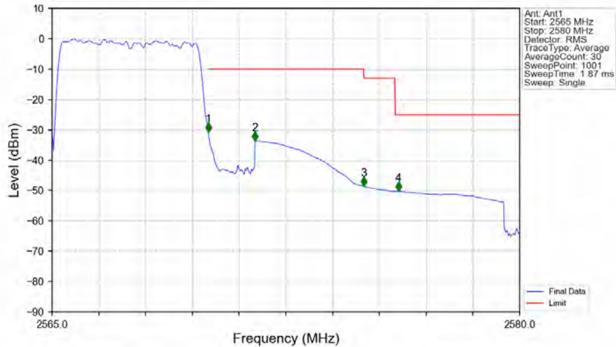
Band7_5MHz_QPSK_HCH_2567.5MHz_RB_25_0_NTNV
