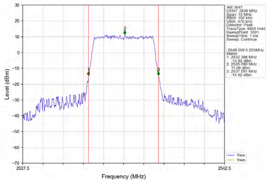
Band7_5MHz_QPSK_MCH_2535MHz_RB_25_0_NTNV
