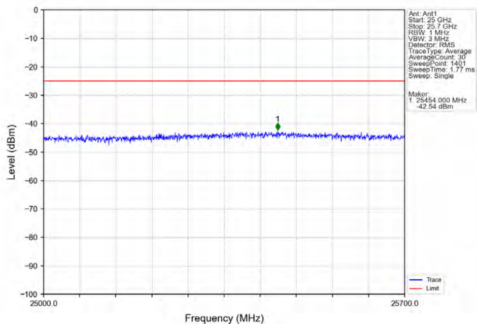
Band7_20MHz_16QAM_HCH_2560MHz_RB_1_99_NTNV
