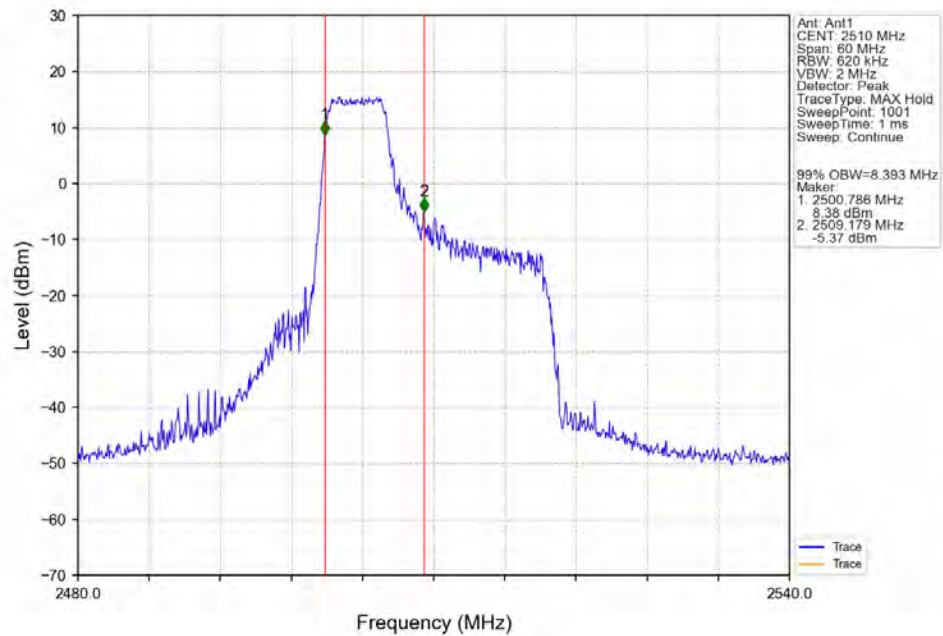
Band7_20MHz_16QAM_LCH_2510MHz_RB_27_0_NTNV
