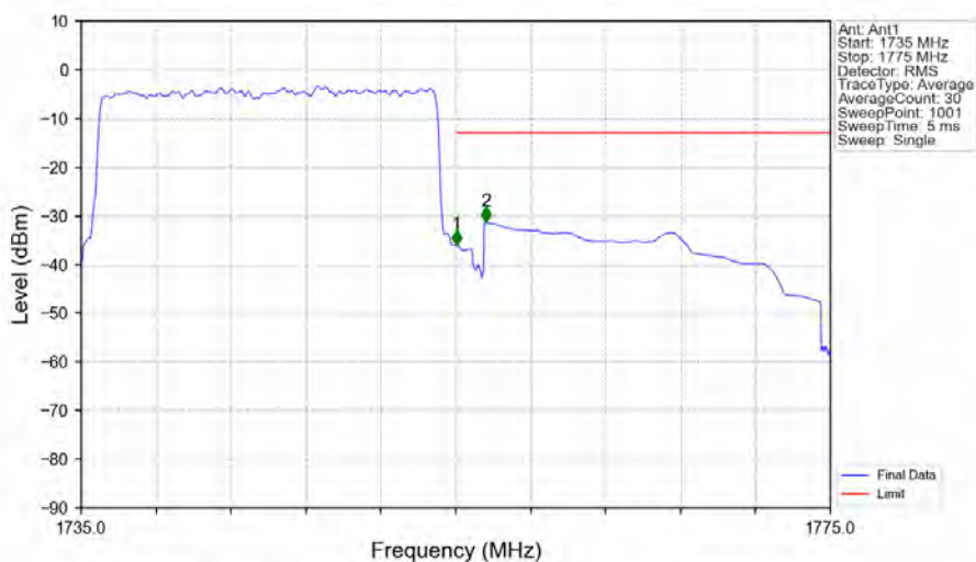
Band4_20MHz_QPSK_HCH_1745MHz_RB_100_0_NTNV
