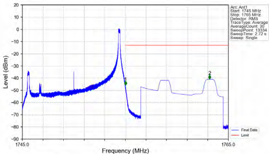
Band4_10MHz_QPSK_HCH_1750MHz_RB_1_49_NTNV
