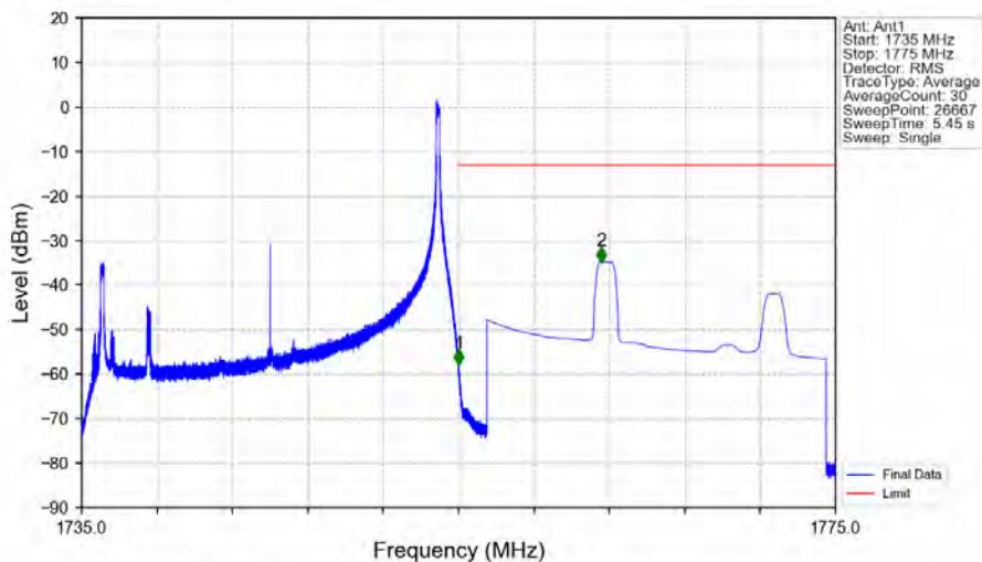
Band4_20MHz_QPSK_HCH_1745MHz_RB_1_99_NTNV
