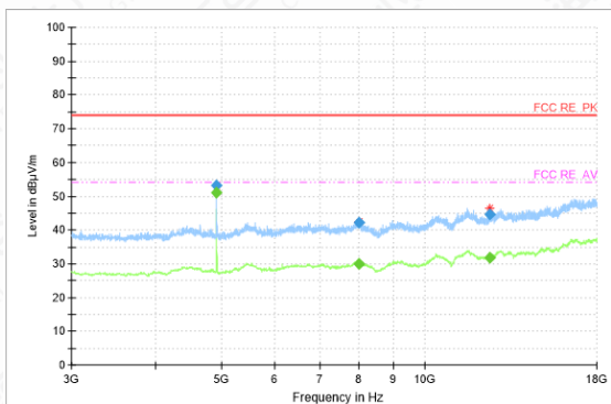
RSE-11B-CH11-3GHz-18GHz
