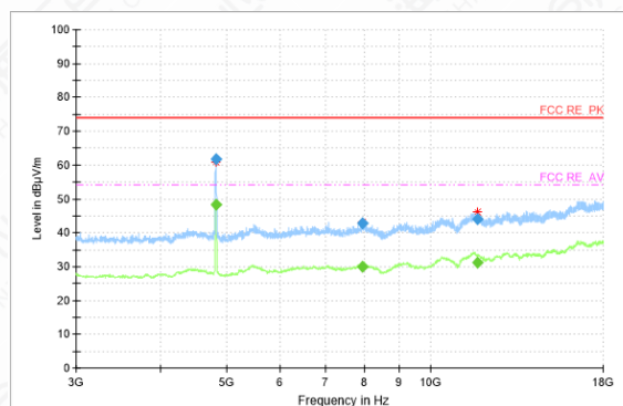
RSE-11G-CH1-3GHz-18GHz
