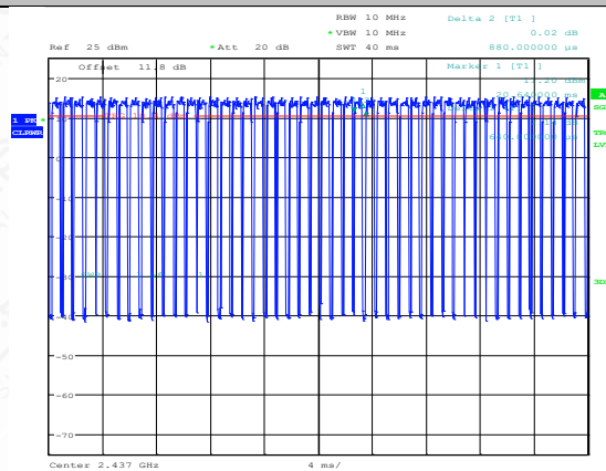
NTNV-11N40MIMO-Ant1-2437
