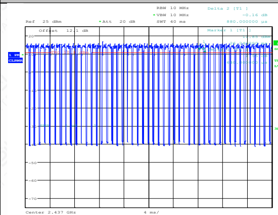
NTNV-11N40MIMO-Ant2-2437
