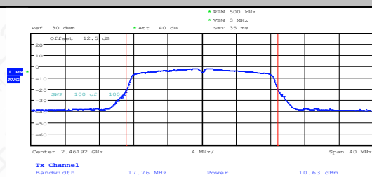
11G-CDD-Ant2-2462-PASS
