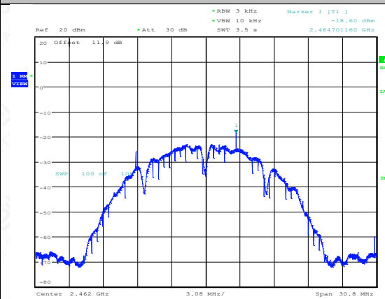
11B-CDD-Ant2-2462-PASS
