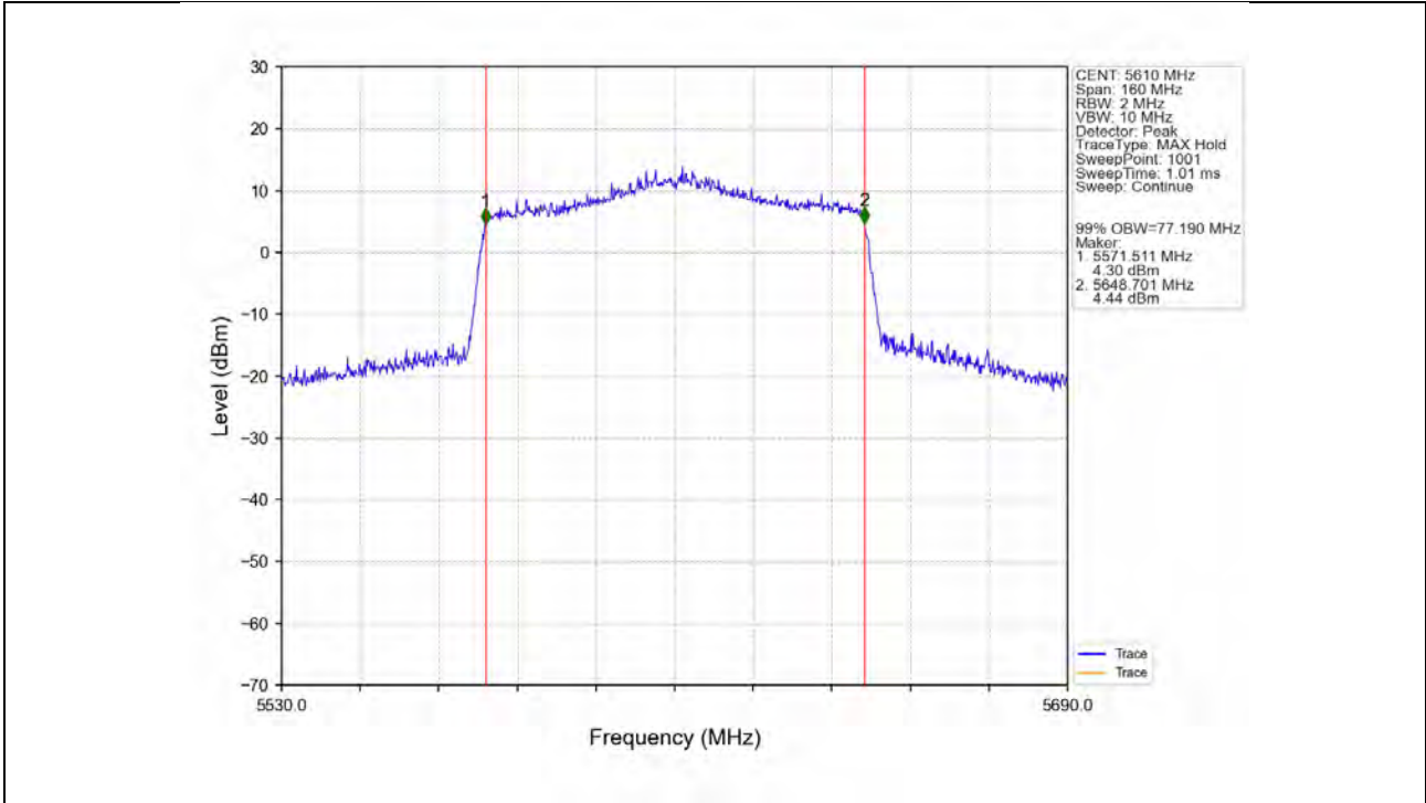
802.11ax(HEW80) HCH_5610MHz_SU / _ANT3_NTNV
