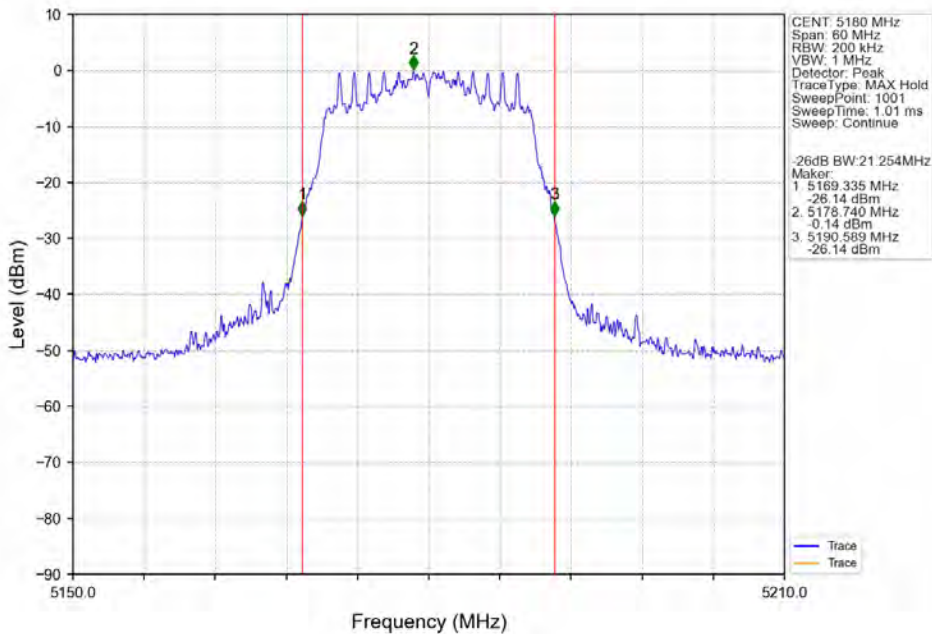
802.11n(HT20)_LCH_5180MHz_ANT3_NTNV
