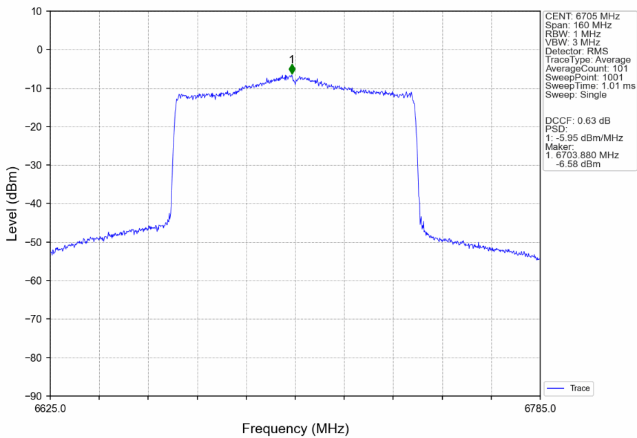
802.11ax(HEW80)_MCH_6705MHz_SU / _ANT2_NTNV
