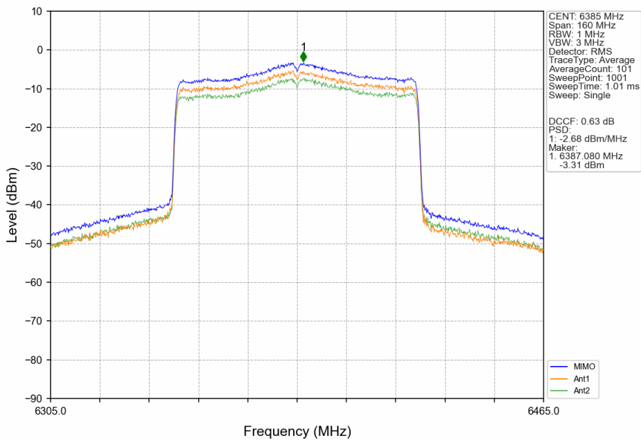
802.11ax(HEW80)_HCH_6385MHz_SU_/_MIMO_NTNV
