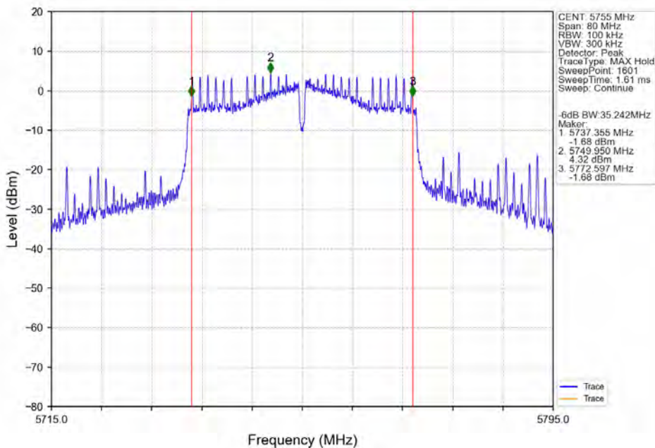
802.11n(HT40)_LCH_5755MHz_ANT3_NTNV
