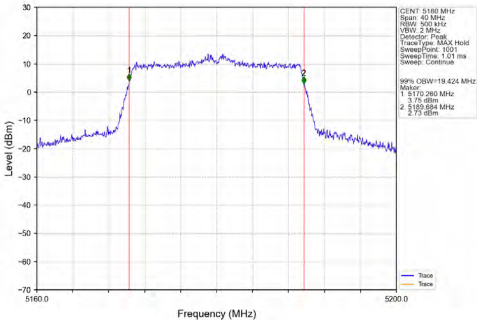
802.11ax(HEW20) LCH 5180MHz_SU / _ANT3_NTNV
