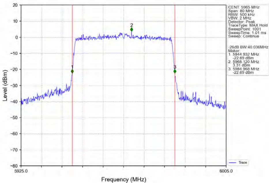
802.11ax(HEW40) LCH 5965MHz SU / ANT3 NTN
