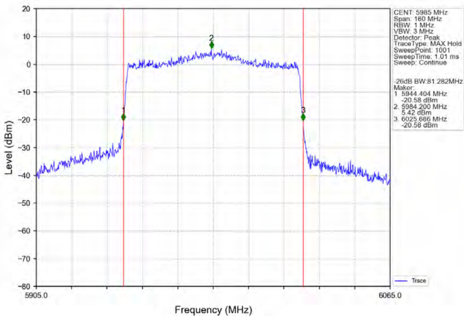
802.11ax(HEW80) LCH 5985MHz SU / ANT3 NTN
