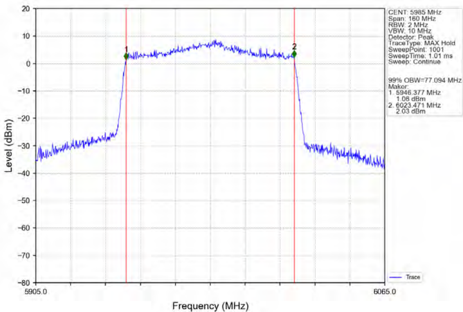
802.11ax(HEW80) LCH 5985MHz SU / ANT3 NTN
