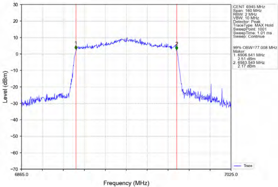
802.11ax(HEW80) LCH 6945MHz SU / ANT3 NTN
