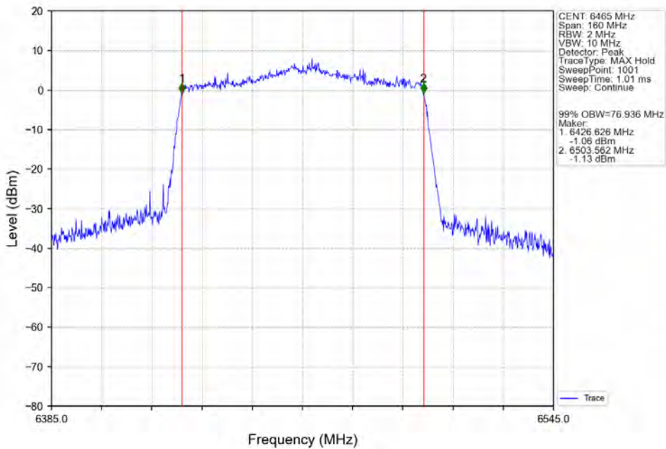
802.11ax(HEW80) LCH 6465MHz SU / ANT3 NTN
