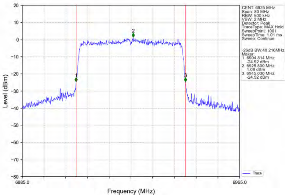
802.11ax(HEW40) LCH 6925MHz SU / ANT3 NTN
