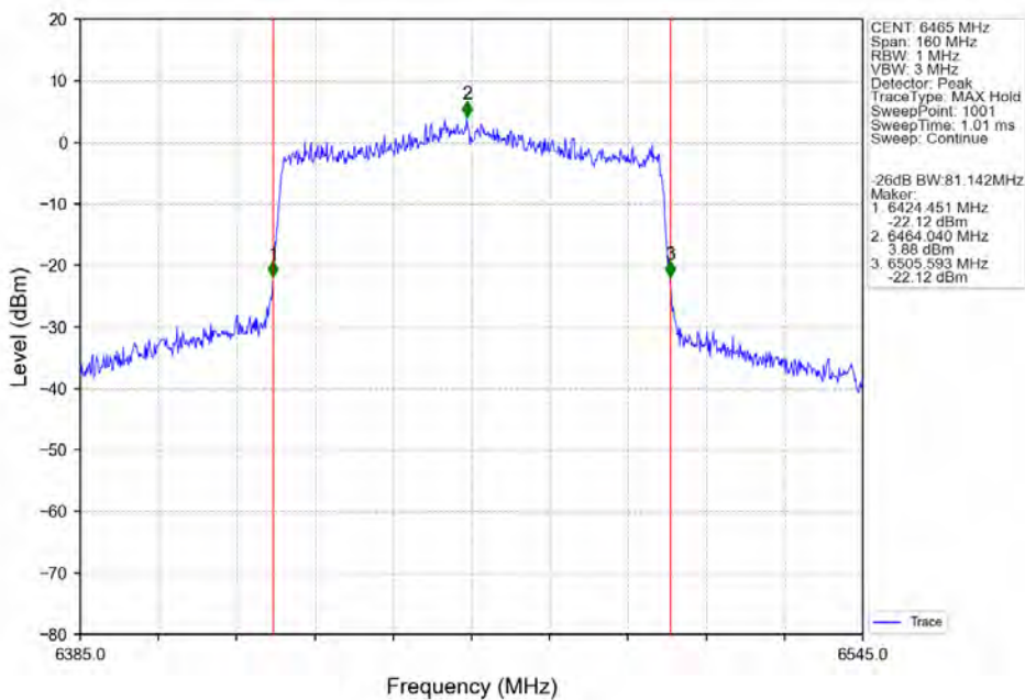
802.11ax(HEW80) LCH 6465MHz SU / ANT3 NTN
