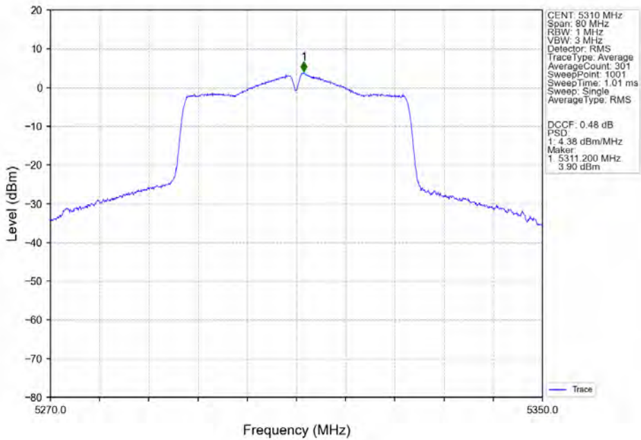
802.11n(HT40) HCH 5310MHz ANT3 NTNv
