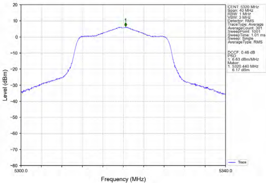
802.11ax(HEW20) HCH 5320MHz SU / ANT2_NTNV
