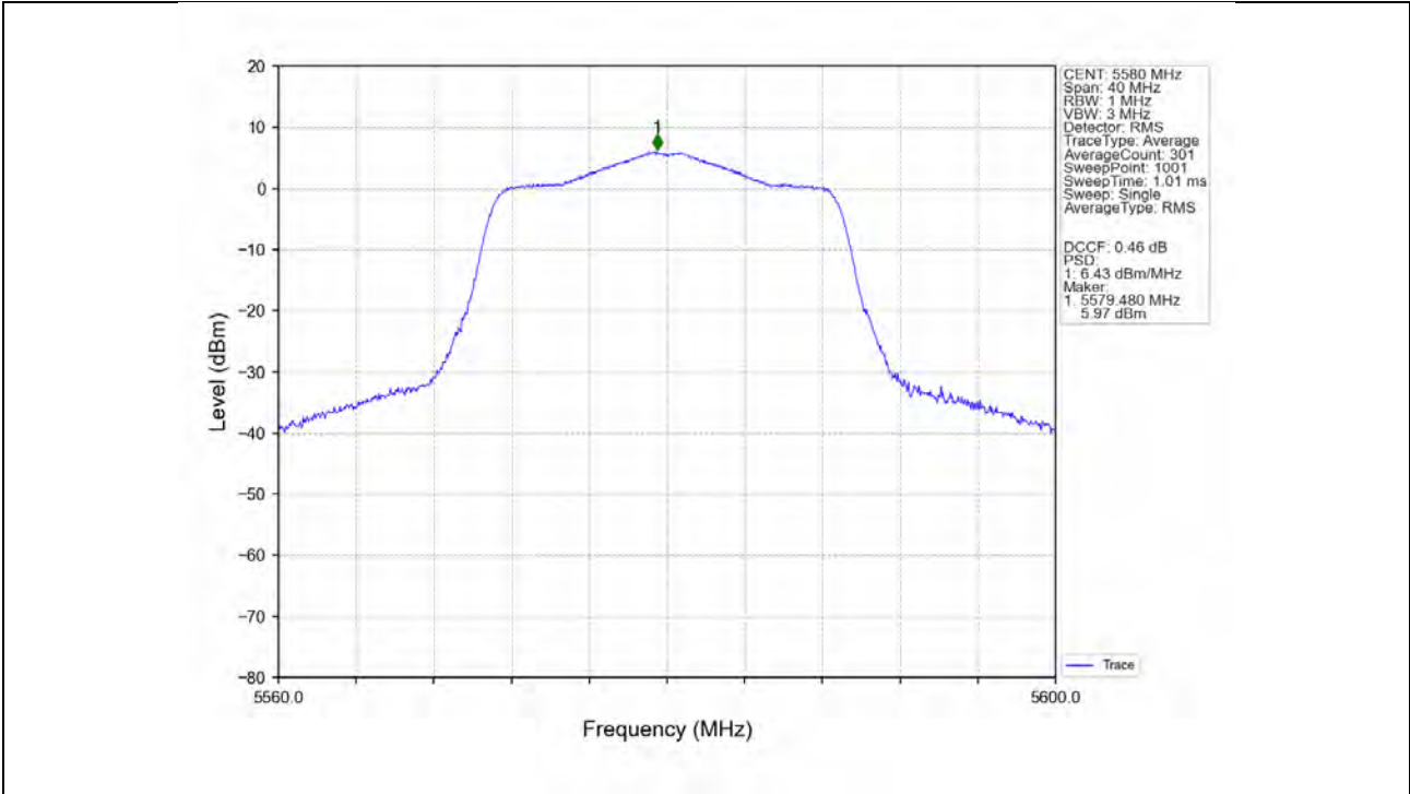
802.11ax(HEW20) MCH 5580MHz SU / MIMO_NTNV
