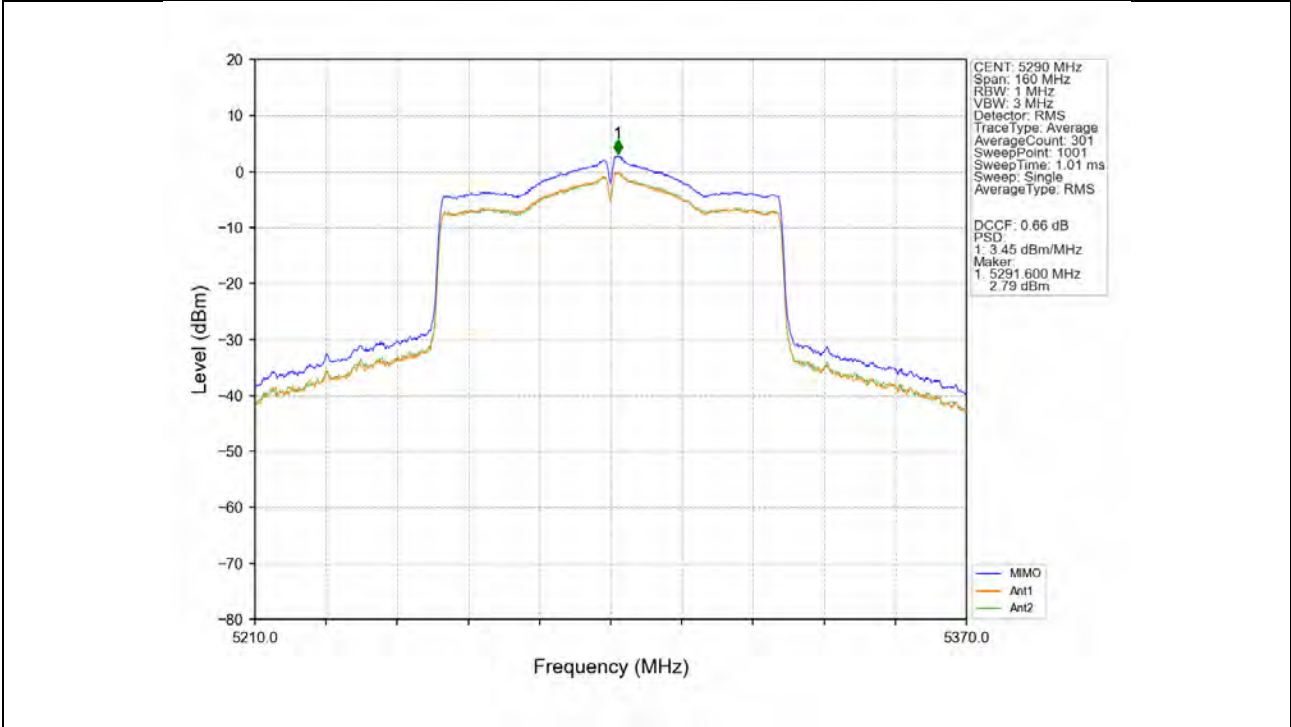
802.11ax(HEW80) MCH 5290MHz SU / MIMO_NTNV
