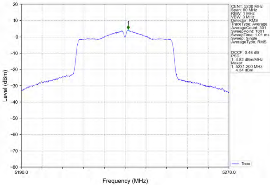
802.11n(HT40)_HCH_5230MHz_ANT3_NTNV
