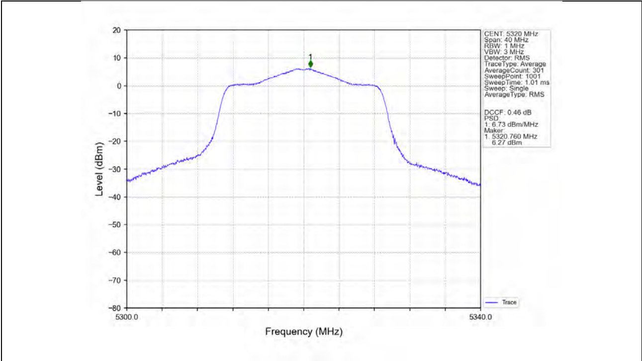
802.11ax(HEW20) HCH 5320MHz SU / MIMO_NTNV
