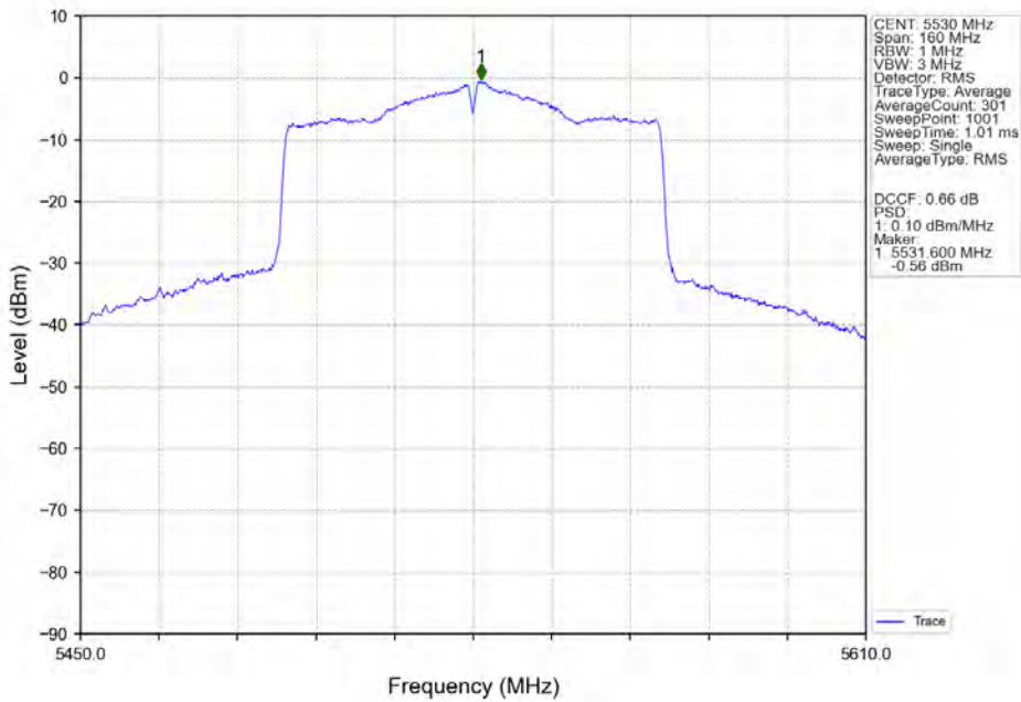
802.11ax(HEW80) LCH 5530MHz SU / ANT3_NTNV
