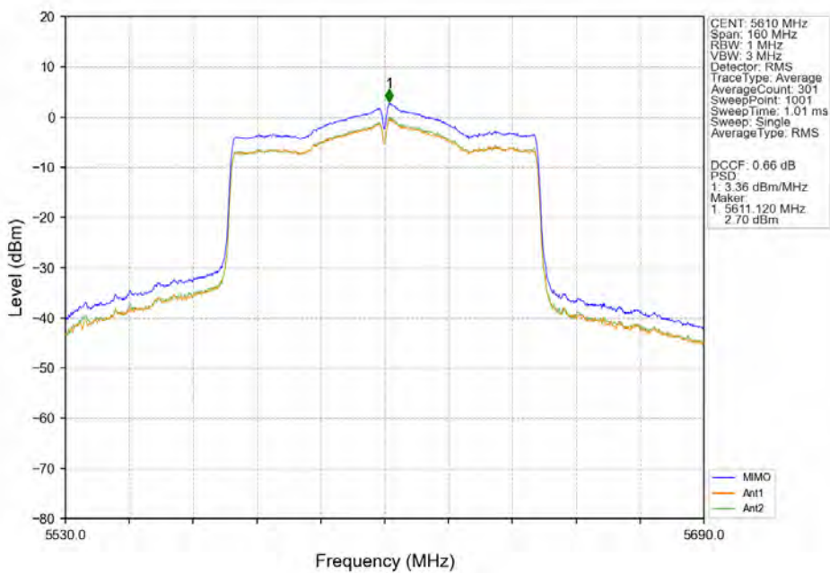
802.11ax(HEW80) HCH_5610MHz_SU_/_MIMO_NTNV
