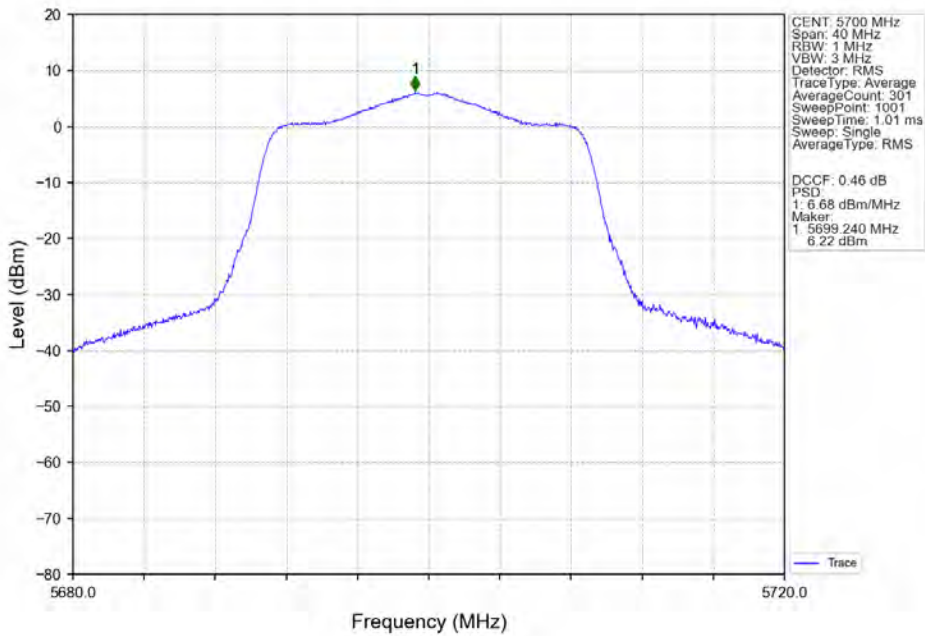
802.11ax(HEW20) HCH 5700MHz SU / _ANT3_NTNV
