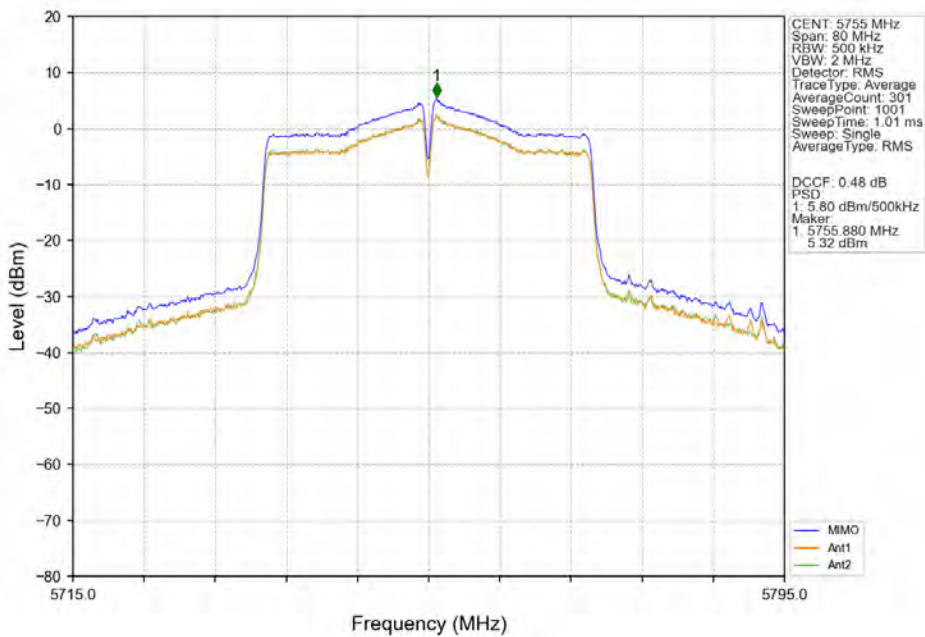
802.11n(HT40)_LCH_5755MHz_MIMO_NTNV
