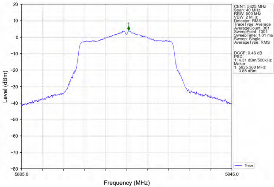
802.11ax(HEW20) HCH 5825MHz SU / _ANT3_NTNV
