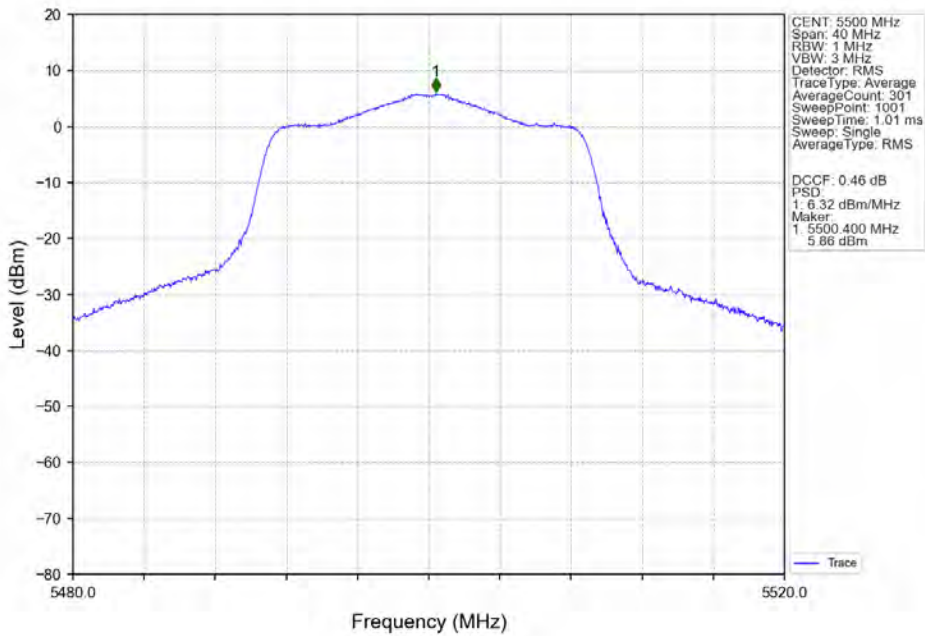
802.11ax(HEW20) LCH 5500MHz SU / _ANT3_NTNV
