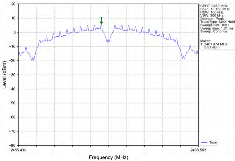
802.11b HCH 2462MHz_Ant3 (SISO) NTN
