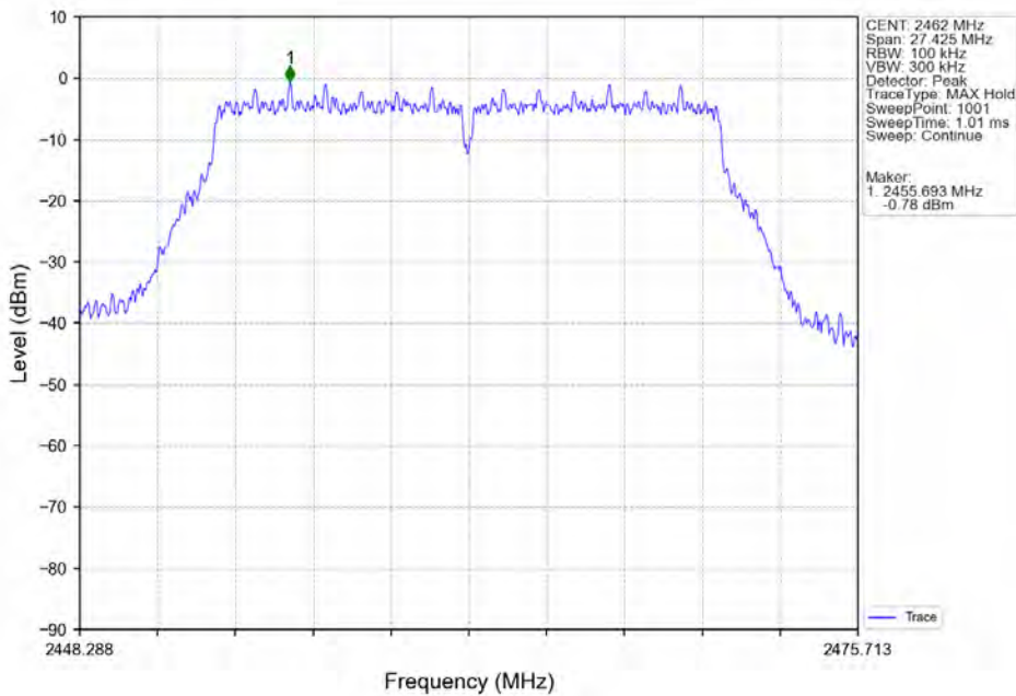
802.11n(HT20) HCH_2462MHz_Ant3 (MIMO)_NTNV
