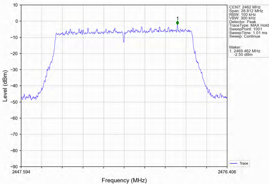
802.11ax(HEW20) HCH 2462MHz SU / Ant3 (MIMO) NTN
