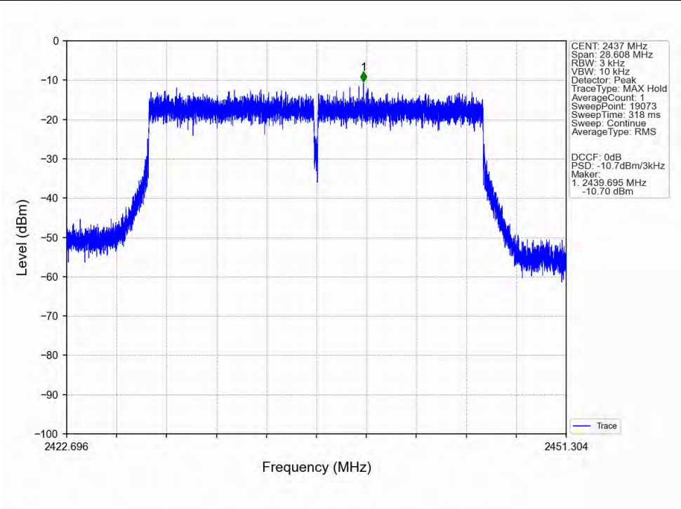
802.11ax(HEW20) MCH_2437MHz_SU / ANT3 (MIMO) NTNv
