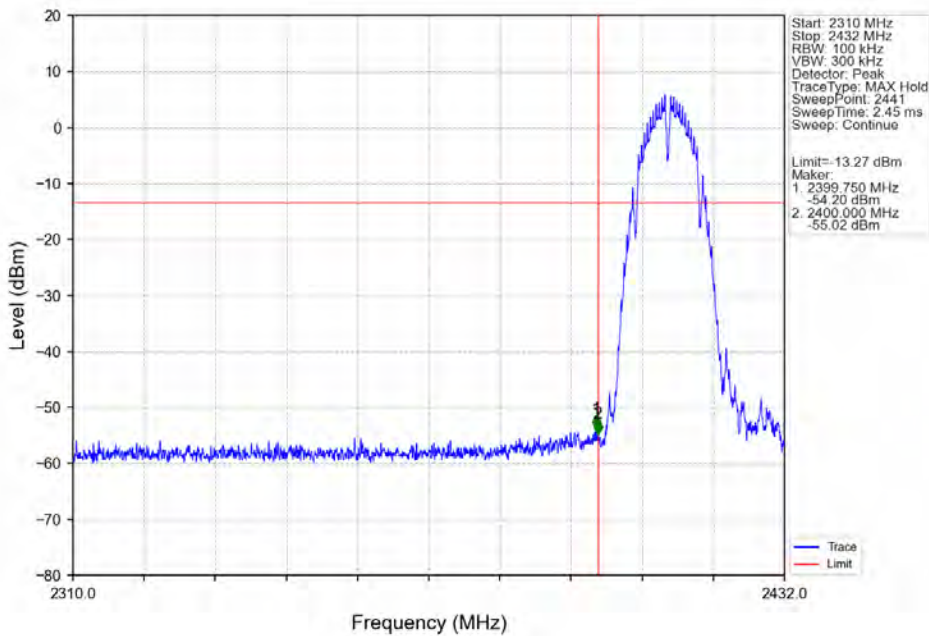
802.11b LCH 2412MHz_Ant3 (SISO) _NTNV
