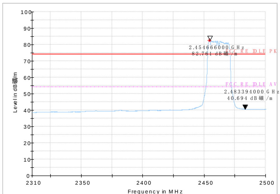
AV detector
