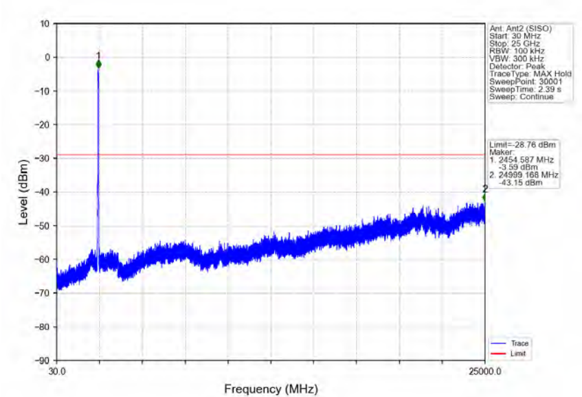
802.11n(HT40)_HCH_2452MHz_Ant2 (SISO)_NTNV
