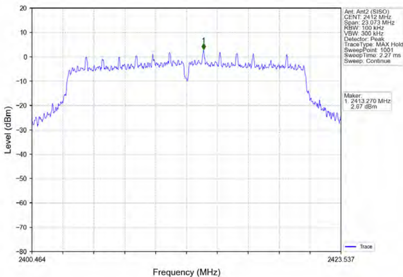
802.11n(HT20)_LCH_2412MHz_Ant2 (SISO)_NTNV
