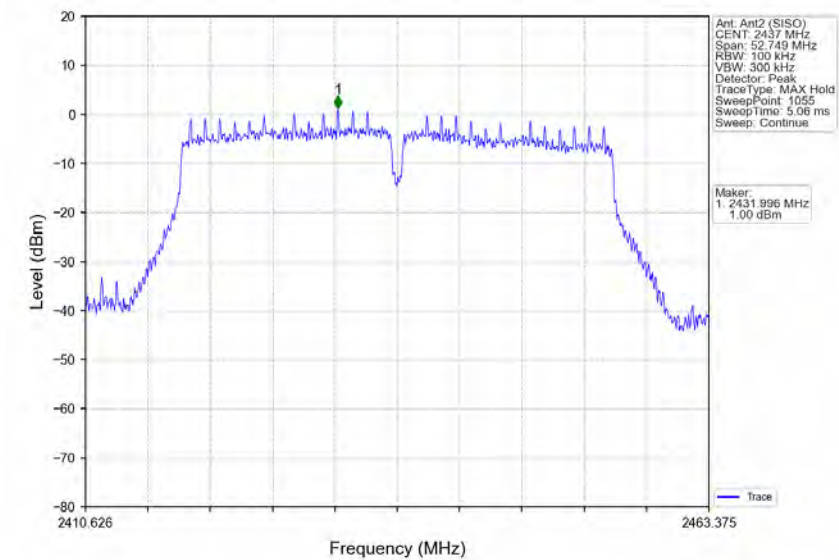
802.11n(HT40)_MCH_2437MHz_Ant2 (SISO)_NTNV
