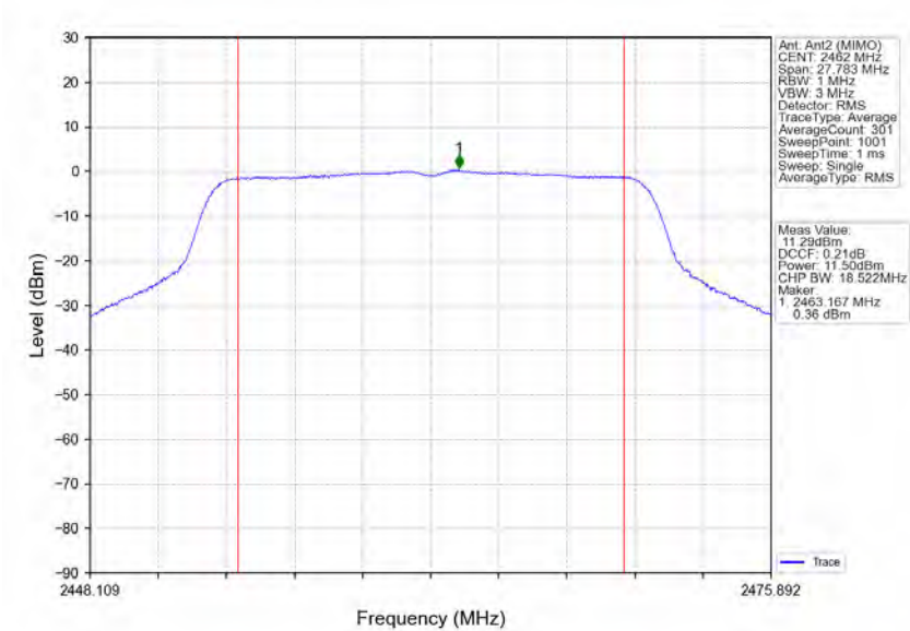
802.11n(HT20)_HCH_2462MHz_Ant2 (MIMO)_NTNV
