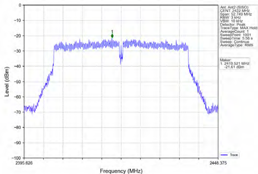
802.11n(HT40)_LCH_2422MHz_Ant2 (SISO)_NTNV
