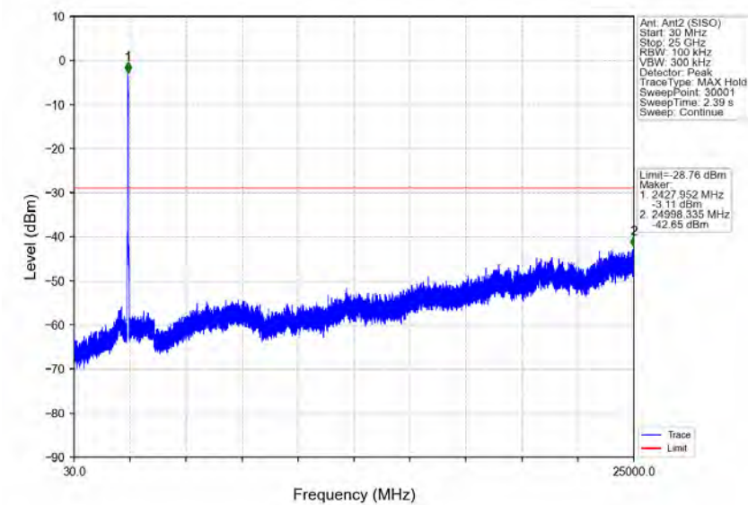
802.11n(HT40)_MCH_2437MHz_Ant2 (SISO)_NTNV
