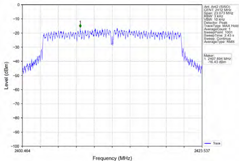
802.11n(HT20)_LCH_2412MHz_Ant2 (SISO)_NTNV
