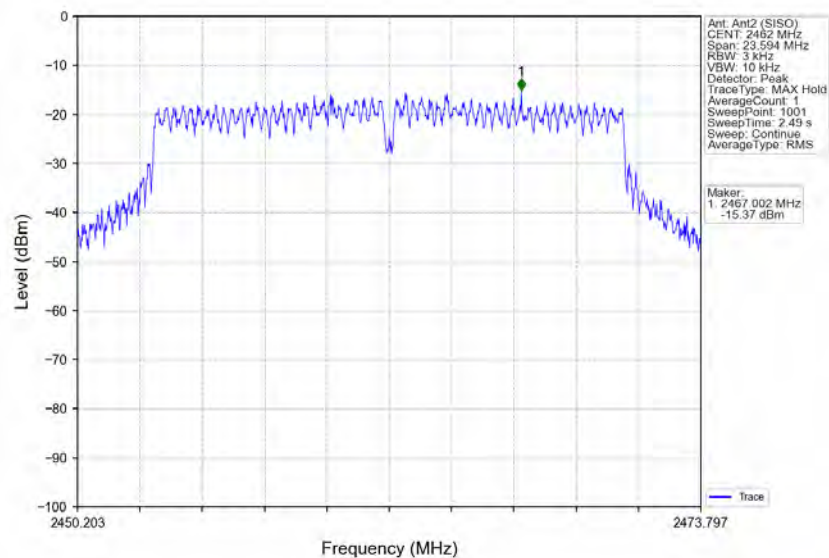
802.11n(HT20)_HCH_2462MHz_Ant2 (SISO)_NTNV
