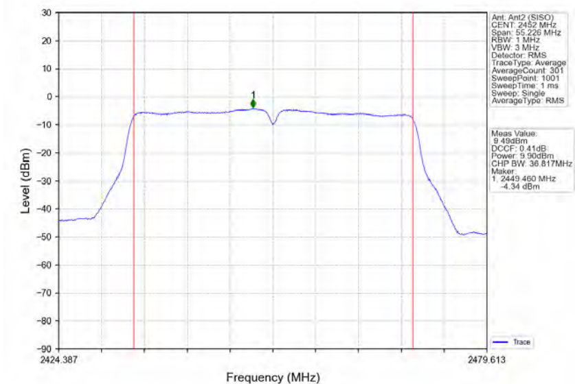
802.11n(HT40)_HCH_2452MHz_Ant2 (SISO)_NTNV
