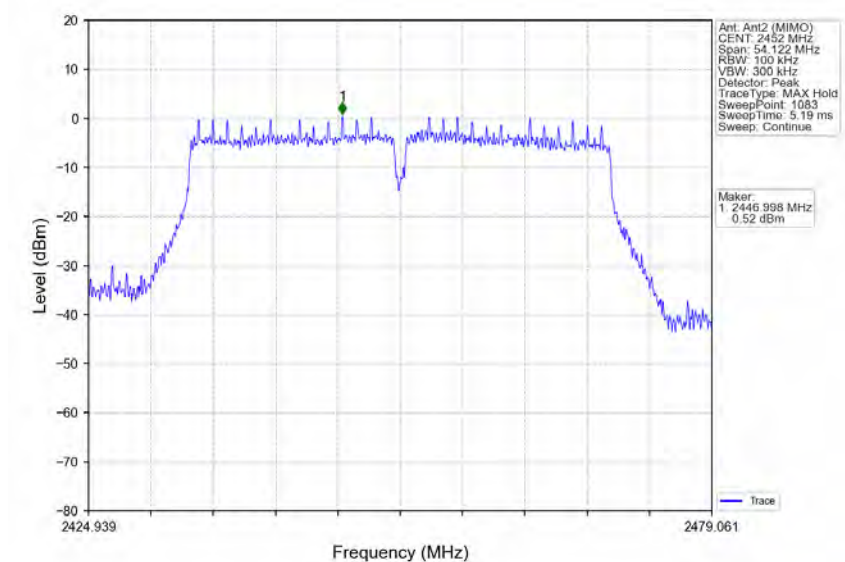
802.11n(HT40)_HCH_2452MHz_Ant2 (MIMO)_NTNV
