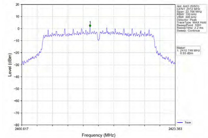
802.11g_LCH_2412MHz_Ant2 (SISO)_NTNV
