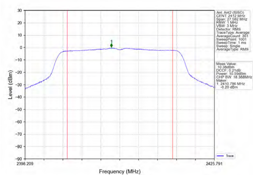
802.11n(HT20)_LCH_2412MHz_Ant2 (SISO)_NTNV
