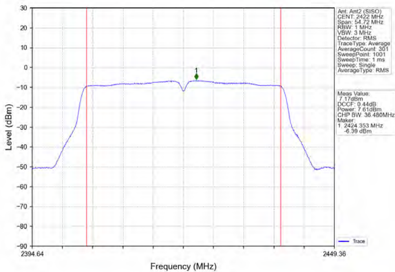
802.11n(HT40)_LCH_2422MHz_Ant2 (SISO)_NTNV
