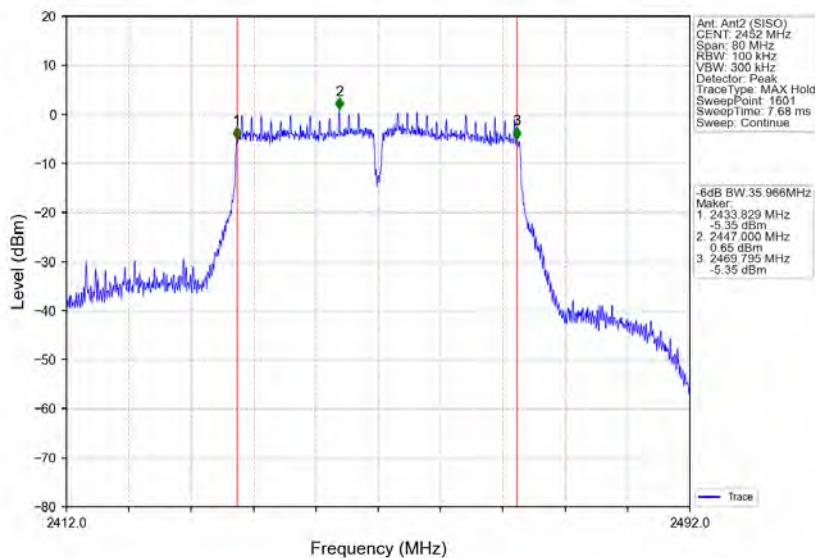
802.11n(HT40)_HCH_2452MHz_Ant2 (SISO)_NTNV
