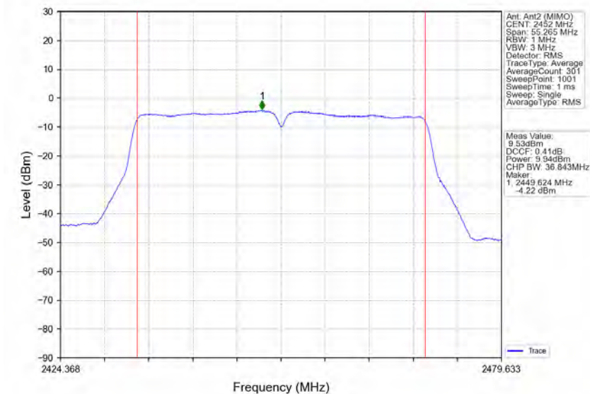
802.11n(HT40)_HCH_2452MHz_Ant2 (MIMO)_NTNV
