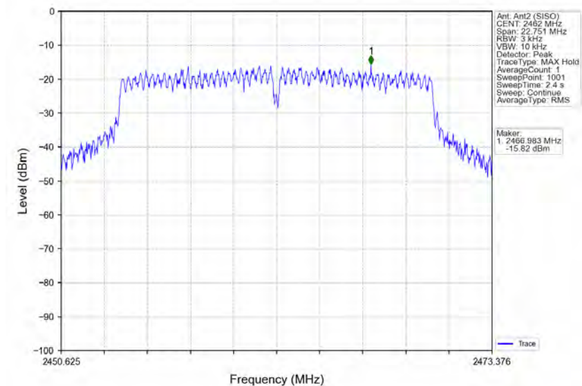
802.11g_HCH_2462MHz_Ant2 (SISO)_NTNV
