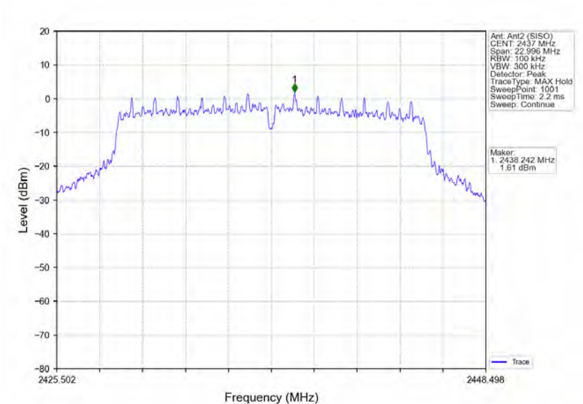
802.11g_MCH_2437MHz_Ant2 (SISO)_NTNV
