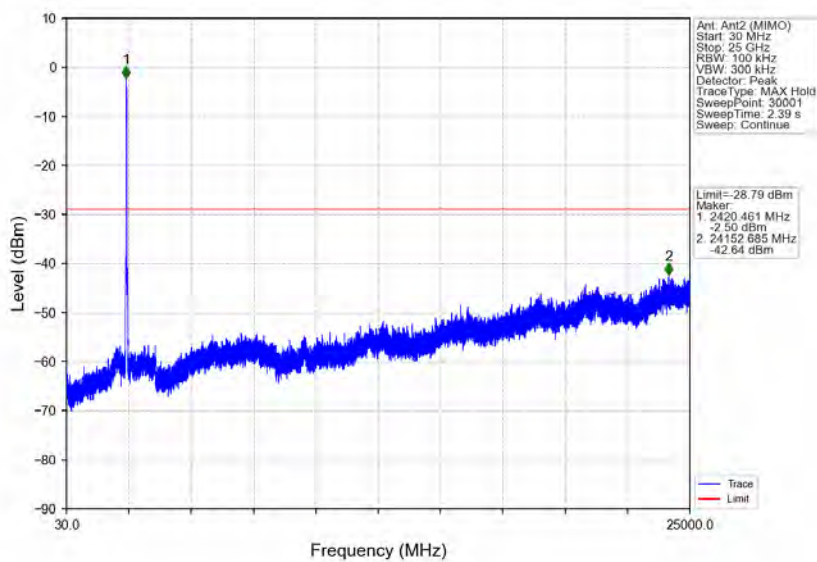
802.11n(HT40)_MCH_2437MHz_Ant2 (MIMO)_NTNV
