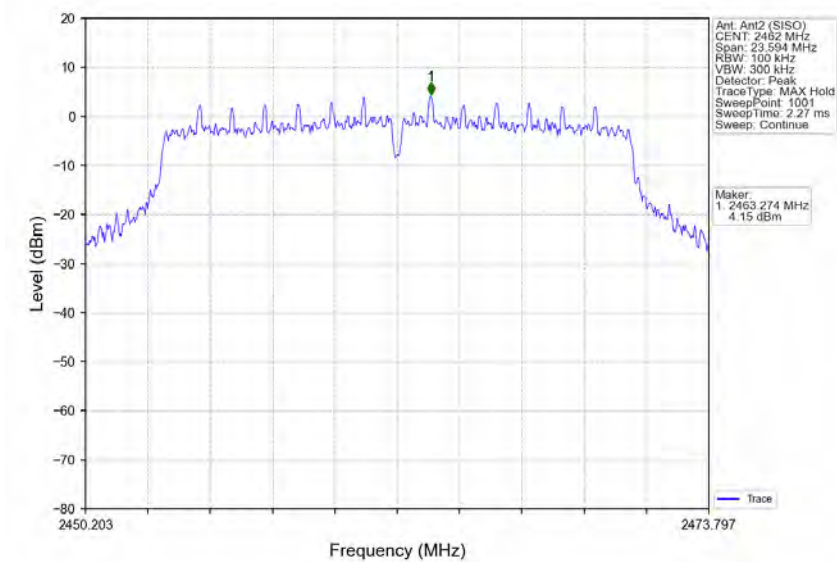
802.11n(HT20)_HCH_2462MHz_Ant2 (SISO)_NTNV
