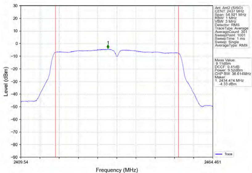
802.11n(HT40)_MCH_2437MHz_Ant2 (SISO)_NTNV
