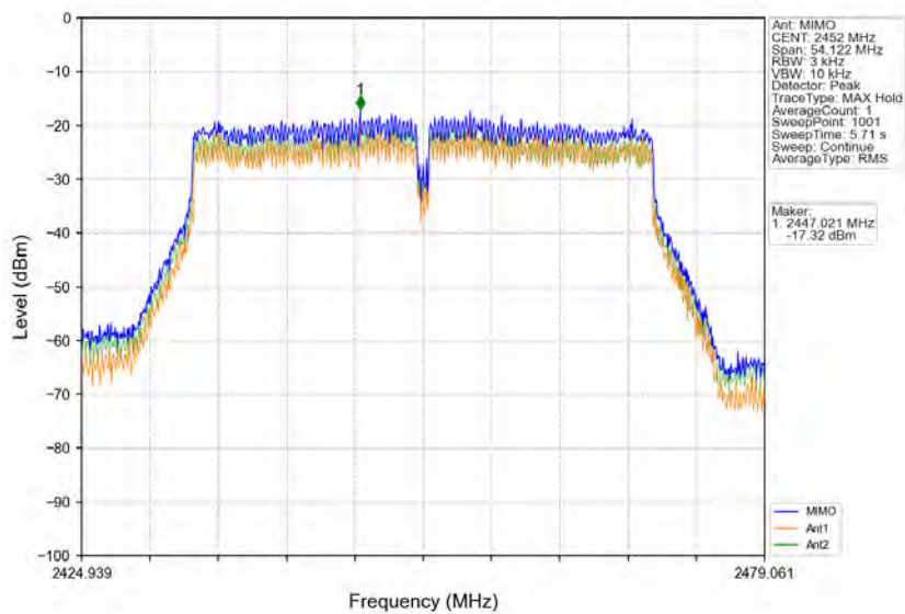
802.11n(HT40)_HCH_2452MHz_MIMO_NTNV
