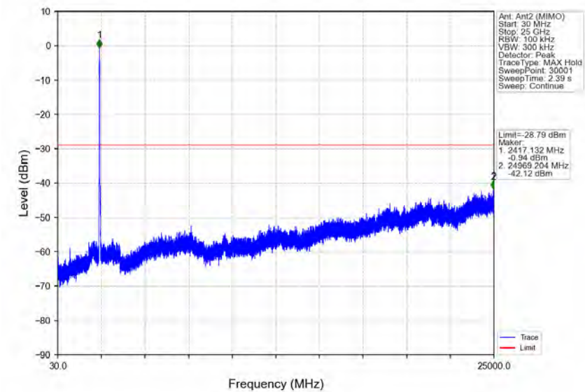
802.11n(HT40)_LCH_2422MHz_Ant2 (MIMO)_NTNV
