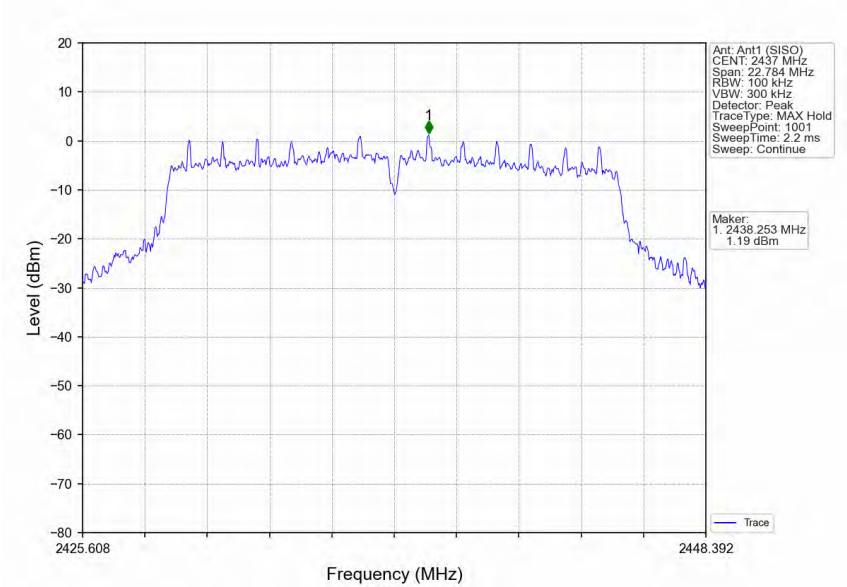
802.11g_MCH_2437MHz_Ant1 (SISO)_NTNV
