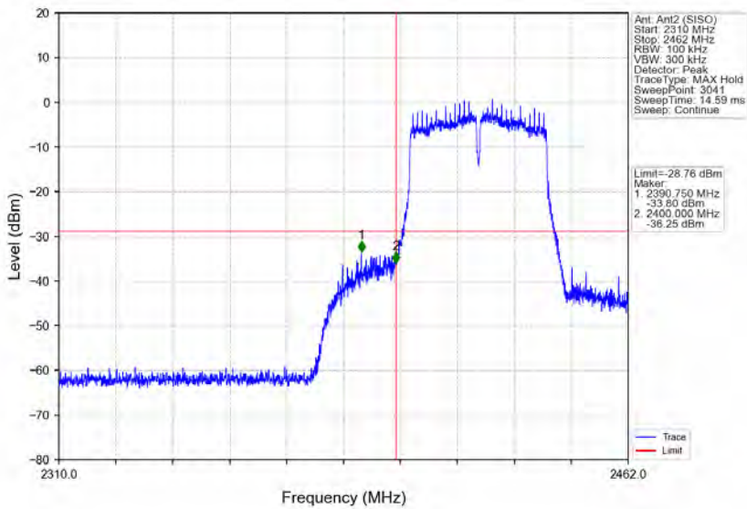
802.11n(HT40)_LCH_2422MHz_Ant2 (SISO)_NTNV
