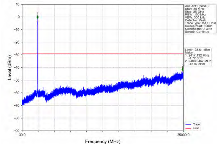
802.11g_LCH_2412MHz_Ant1 (SISO)_NTNV
