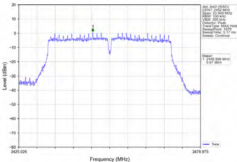
802.11n(HT40)_HCH_2452MHz_Ant2 (SISO)_NTNV
