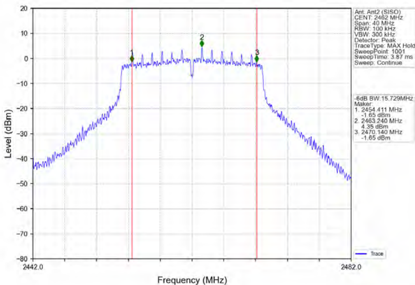
802.11n(HT20)_HCH_2462MHz_Ant2 (SISO)_NTNV
