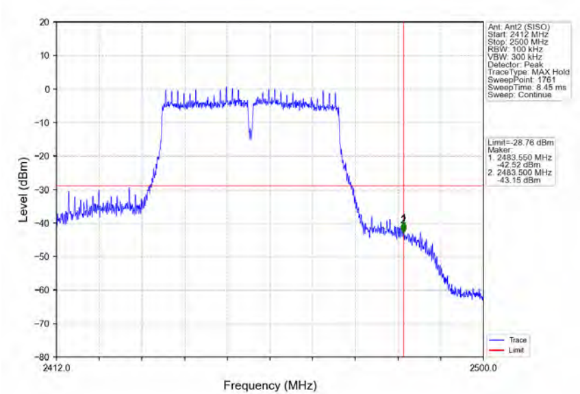
802.11n(HT40)_HCH_2452MHz_Ant2 (SISO)_NTNV
