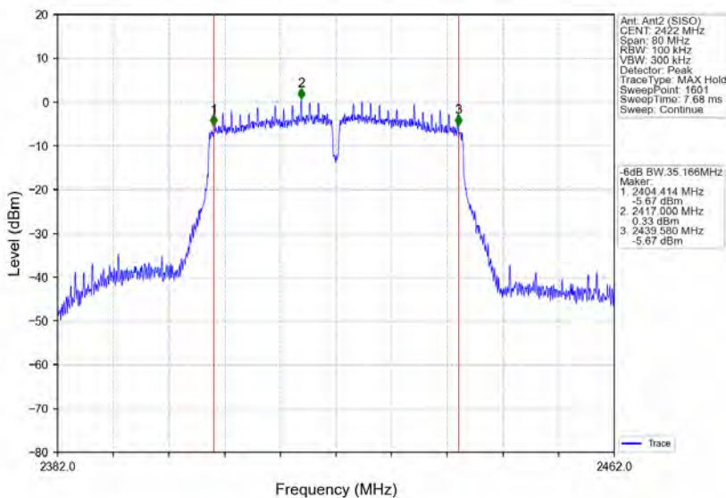
802.11n(HT40)_LCH_2422MHz_Ant2 (SISO)_NTNV
