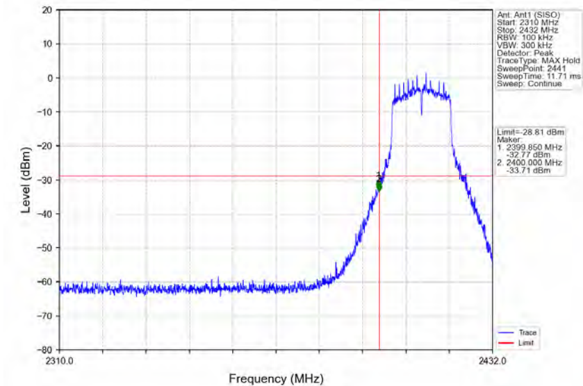
802.11g_LCH_2412MHz_Ant1 (SISO)_NTNV
