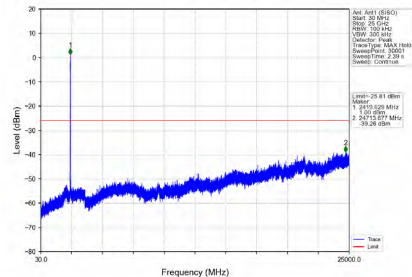
802.11n(HT20)_LCH_2412MHz_Ant1 (SISO)_NTNV
