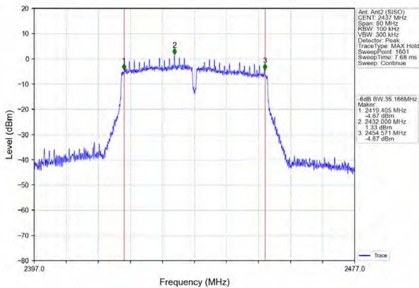
802.11n(HT40)_MCH_2437MHz_Ant2 (SISO)_NTNV
