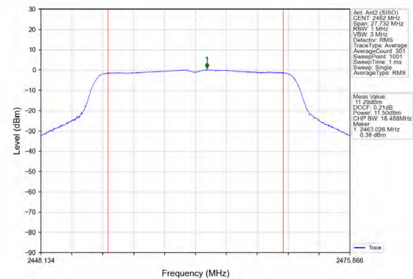
802.11n(HT20)_HCH_2462MHz_Ant2 (SISO)_NTNV
