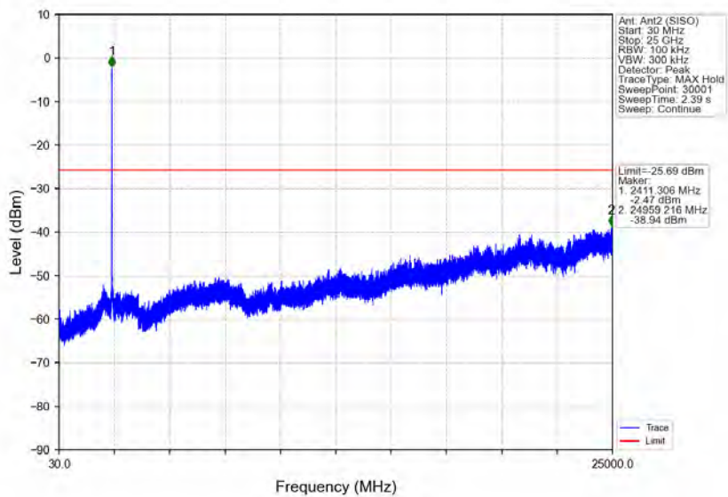
802.11n(HT20)_LCH_2412MHz_Ant2 (SISO)_NTNV
