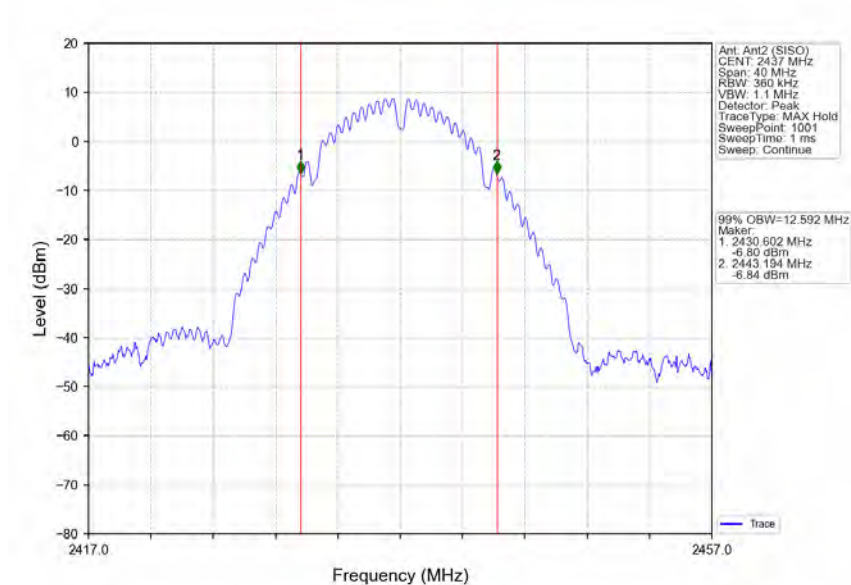
802.11b_MCH_2437MHz_Ant2 (SISO)_NTNV
