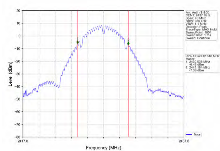
802.11b_MCH_2437MHz_Ant1 (SISO)_NTNV
