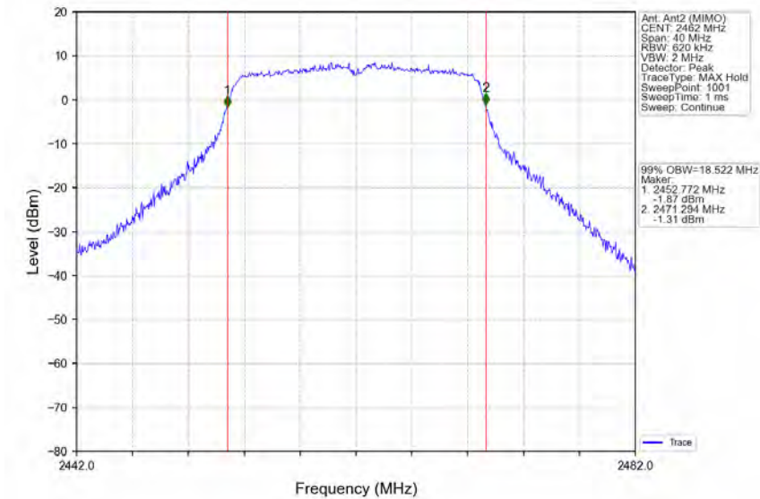
802.11n(HT20)_HCH_2462MHz_Ant2 (MIMO)_NTNV
