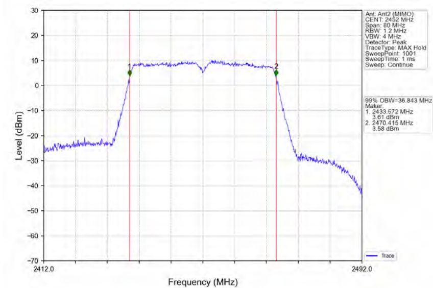
802.11n(HT40)_HCH_2452MHz_Ant2 (MIMO)_NTNV
