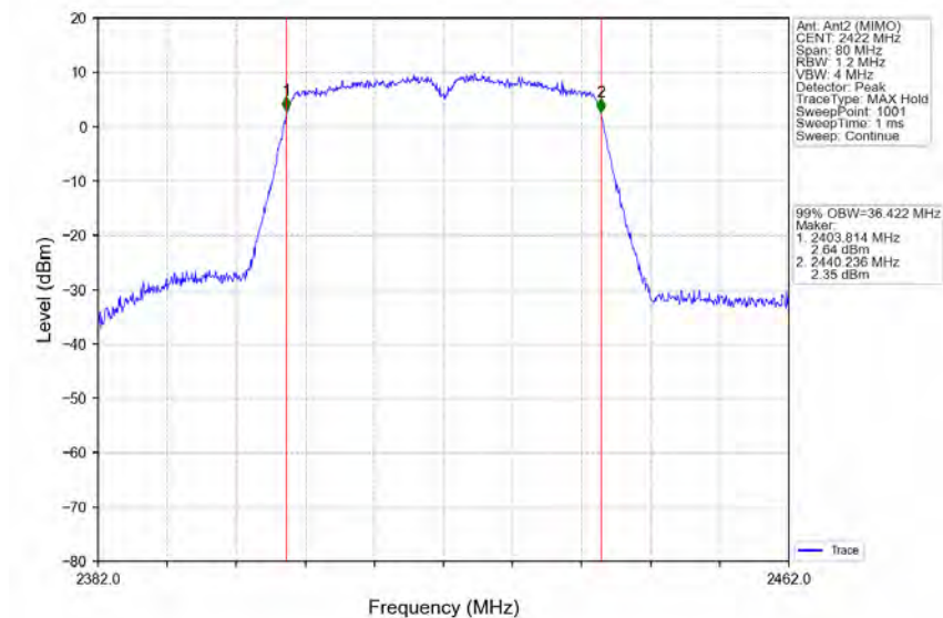
802.11n(HT40)_LCH_2422MHz_Ant2 (MIMO)_NTNV
