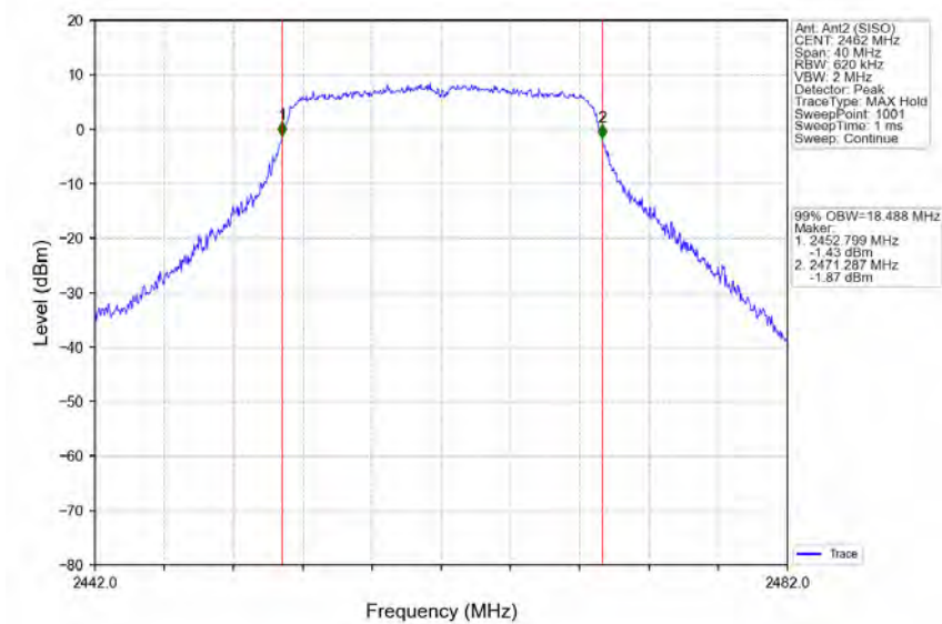
802.11n(HT20)_HCH_2462MHz_Ant2 (SISO)_NTNV
