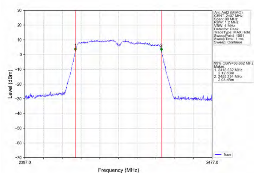
802.11n(HT40)_MCH_2437MHz_Ant2 (MIMO)_NTNV
