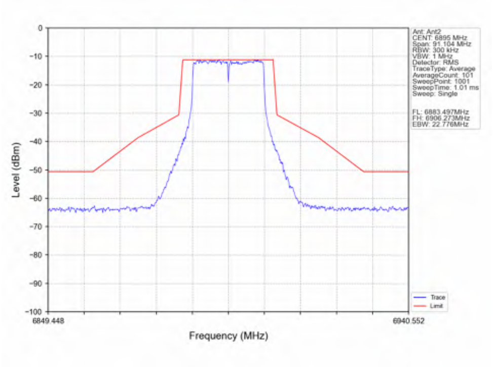
802.11ac(VHT20) LCH_6895MHz_Ant2_NTNV
