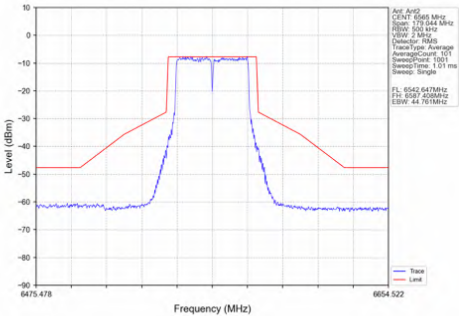
802.11ac(VHT40) LCH_6565MHz_Ant2_NTNV
